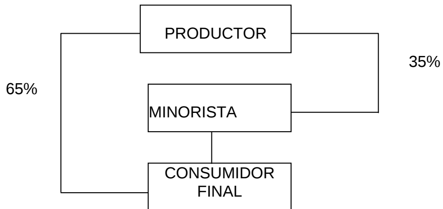
Gráfica 4 Municipio de Colomba, Departamento de Quetzaltenango Canal de Comercialización Actual Miel de Abeja Año: 2001
