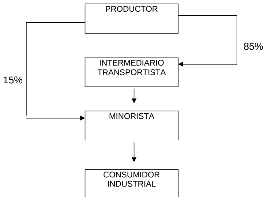
Gráfica 1 Municipio de Colomba, Departamento de Quetzaltenango Canales de Comercialización Café Cereza Microfincas y Fincas Sub-familiares Año: 2001
