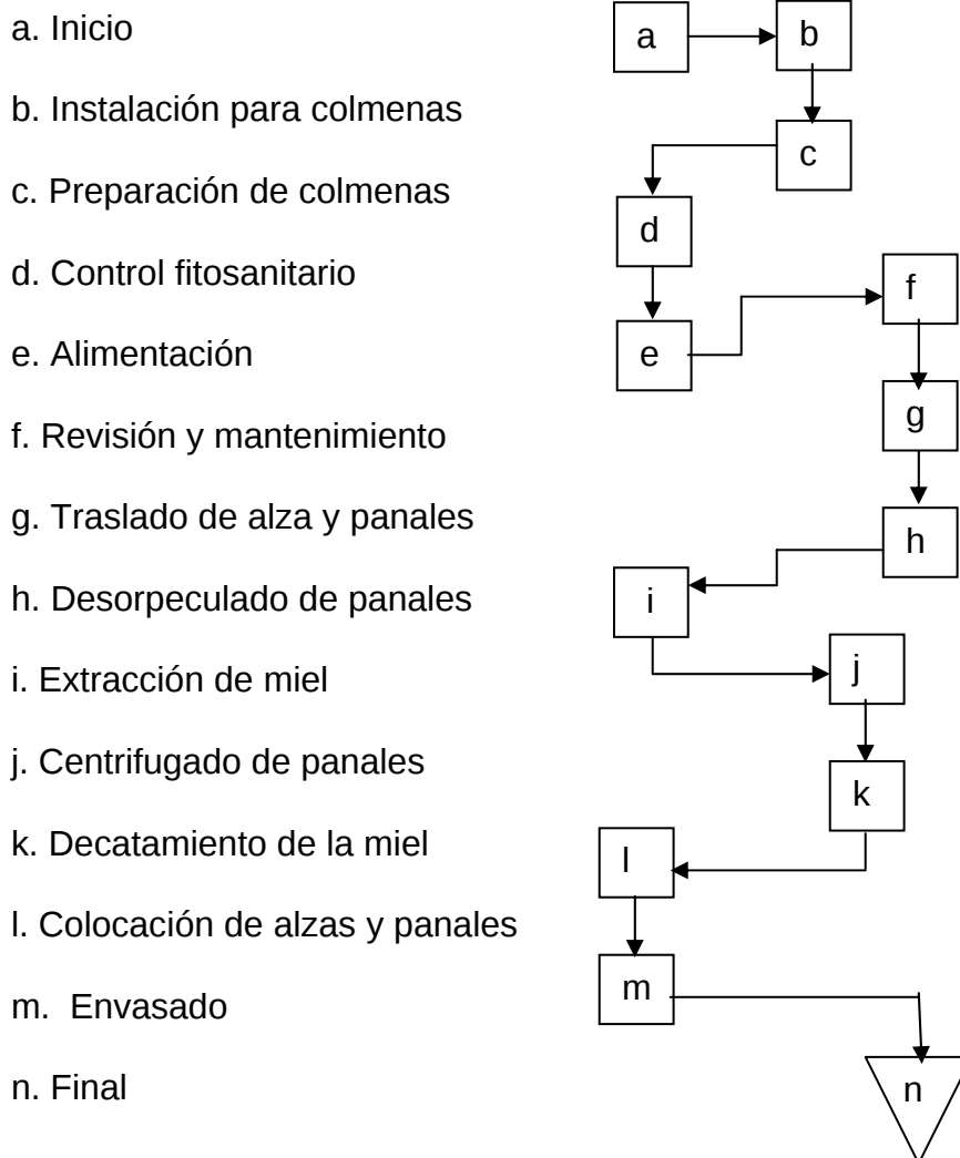
Gráfica 3 Municipio de Colomba, Departamento de Quetzaltenango Proyecto: Producción de Miel de Abeja Flujograma del Proceso Productivo Año: 2001
