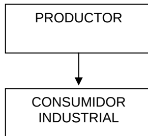
Gráfica 2 Municipio de Colimba, Departamento de Quetzaltenango Canales de Comercialización Café Pergamino Fincas Familiares y Multifamiliares Año: 2001
