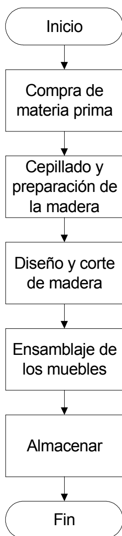
Gráfica 6 Aldea El Zapote, Municipio de San Pedro Pinula - Jalapa Proyecto: Asociación de Artesanos Productores de Muebles de Madera Flujograma de Proceso de Producción Año 2002
