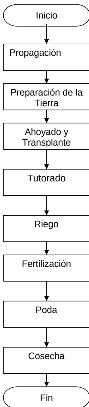
Gráfica 6 Municipio de Monjas, Departamento de Jalapa Proyecto: Producción de Mango de Pashte Diagrama del Proceso Productivo Año: 2003
