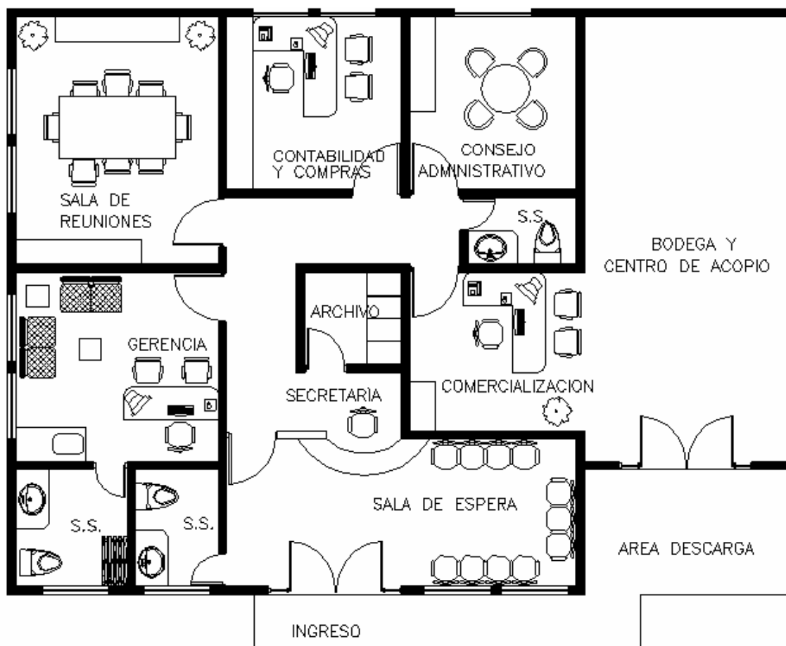
Gráfica 10 Municipio de Monjas, Departamento de Jalapa Proyecto: Producción de Mango de Pashte Distribución en Planta Asociación Agrícola de Productores de Mango de Monjas, Jalapa Año: 2003
