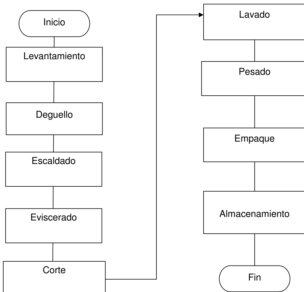
Gráfica 5 Municipio de San Luis Jilotepeque –Jalapa Proyecto: Producción de Carne de Pollo Diagrama del Proceso del Faenado Año 2002
