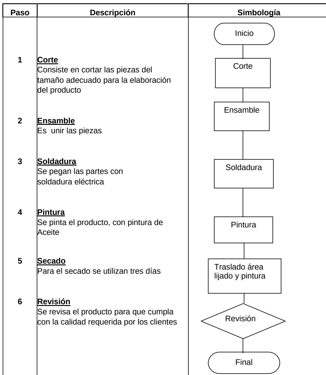
Gráfica 37 Municipio de Santa Bárbara - Huehuetenango Diagrama de Procesos de Elaboración, Rama Herrería Año: 2003
