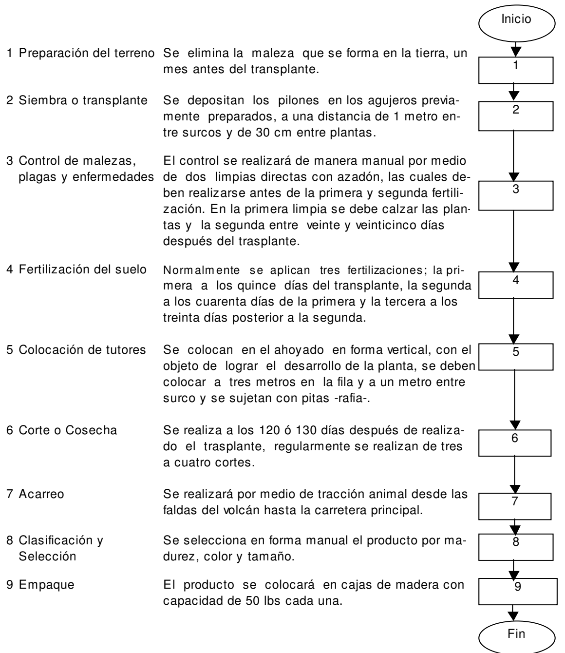
Gráfica 4 Municipio de Santa Catarina Mita – Jutiapa Proyecto: producción de chile pimiento Flujograma del Proceso Productivo del Cultivo de Chile Pimiento Año 2002
