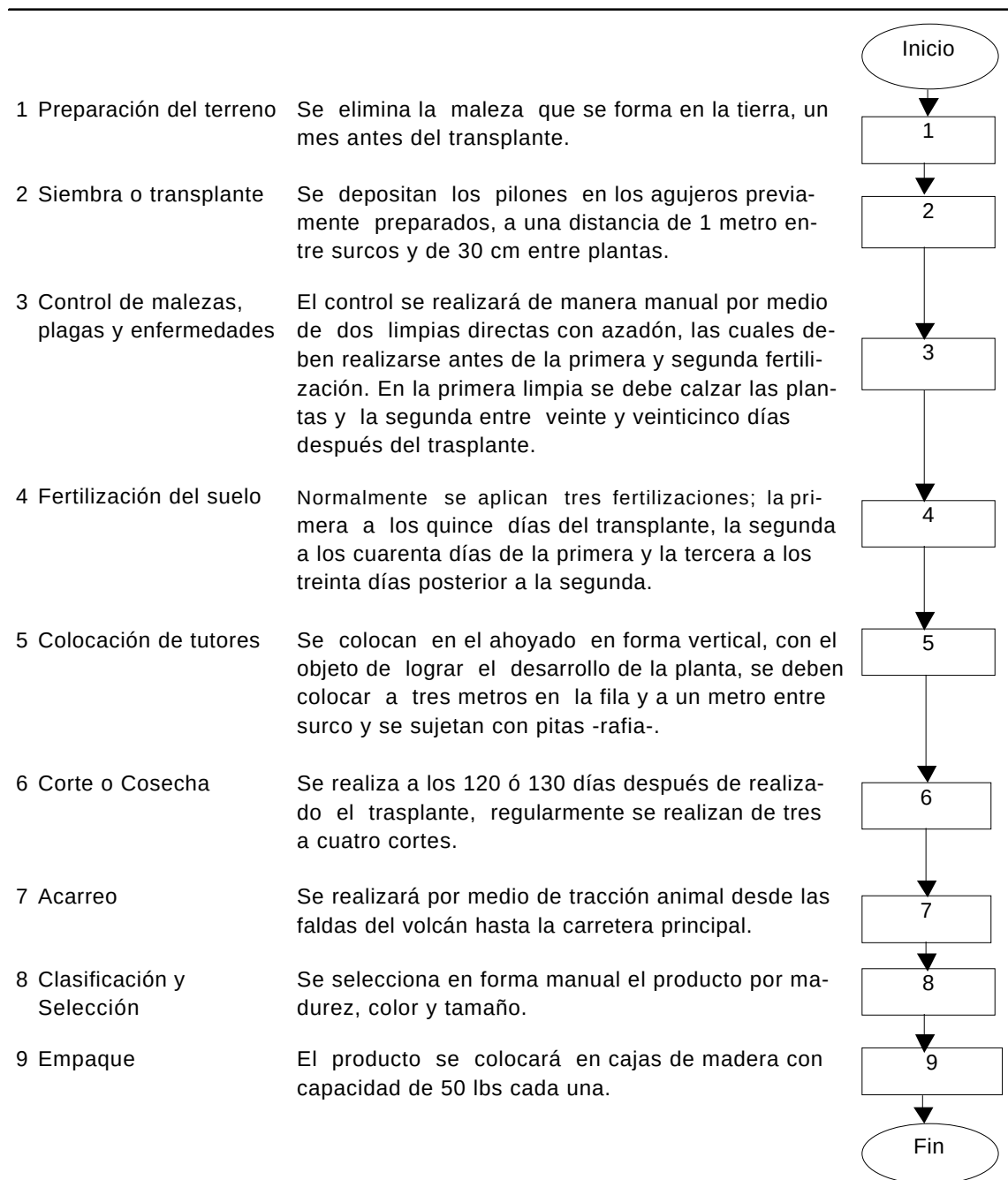
Gráfica 8 Aldea Suchitán, Santa Catarina Mita - Jutiapa Proyecto producción de tomate Flujograma del proceso productivo Año 2002
