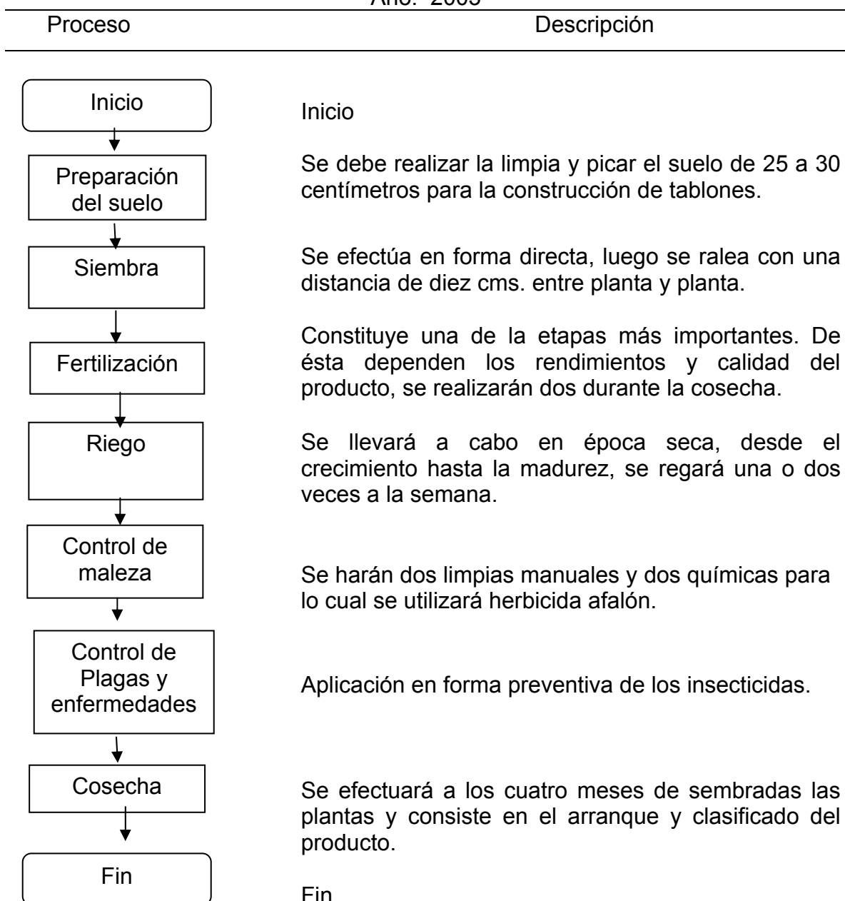
Gráfica 5 Aldea Chisté Municipio de Tectitán, Huehuetenango Proyecto: Producción de Zanahoria Diagrama de Flujo del Proceso Productivo Año: 2003
