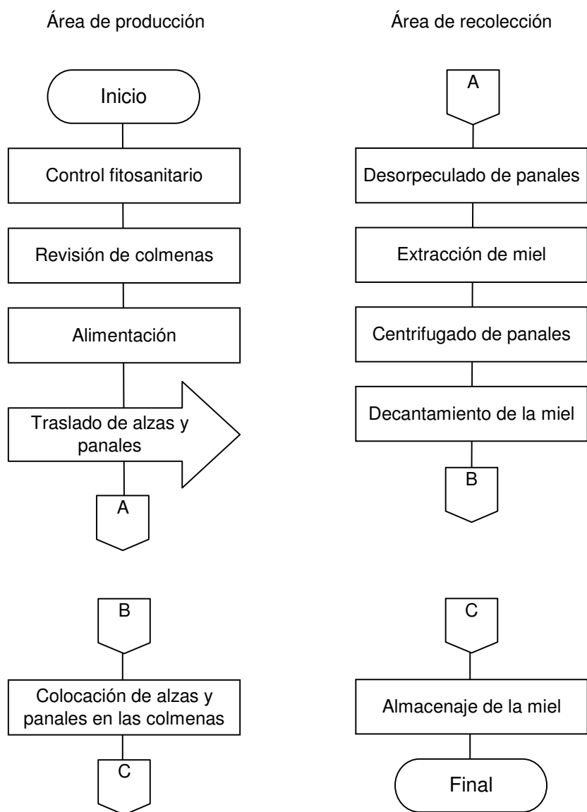
Gráfica 5 Santa Ana Huista - Huehuetenango Proyecto: Producción de Miel de Abeja Diagrama del Proceso Productivo
