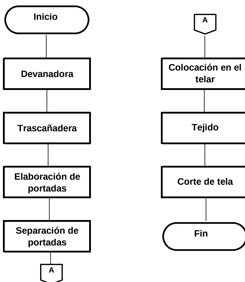
Gráfica 4 Municipio de Concepción Huista - Huehuetenango Flujograma del proceso de producción de tejidos típicos Pequeño artesano Año 2004
