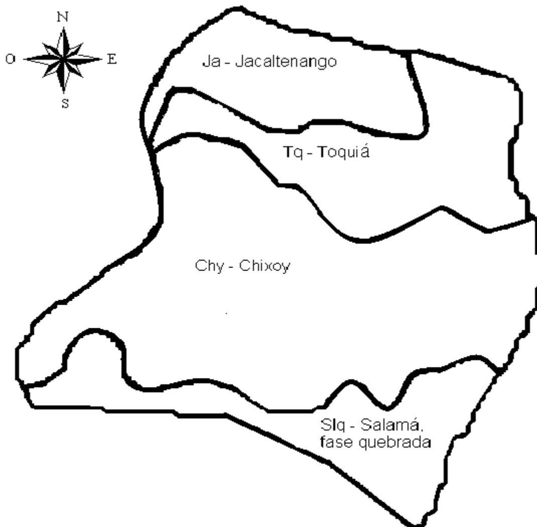
Mapa 7 Municipio de San Sebastián Huehuetenango, Huehuetenango Series de Suelos
