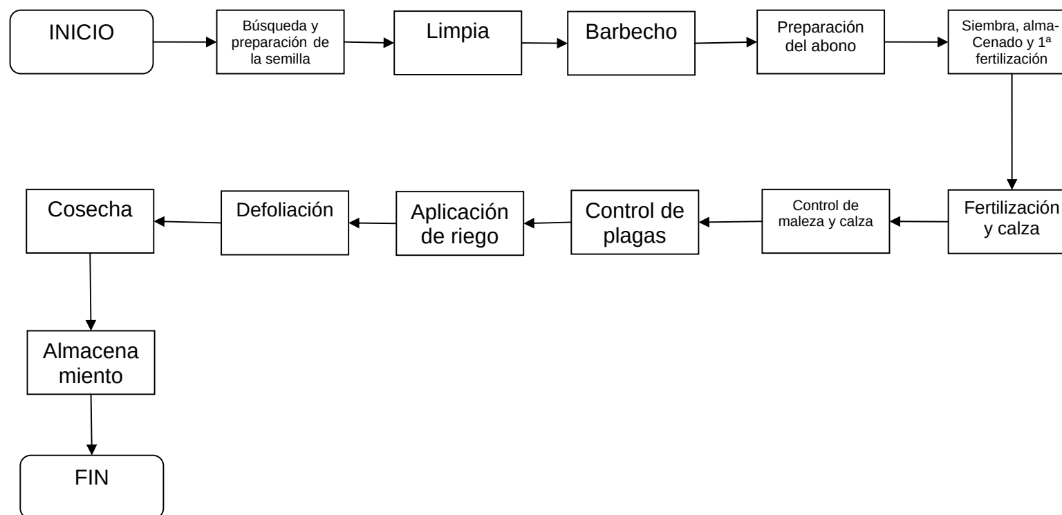
Gráfica 3 Municipio de San Juan Ostuncalco, Departamento de Quetzaltenango Flujo del Proceso Productivo Nivel Tecnológico Tradicional Microfincas Cultivo de Papa Año: 2005
