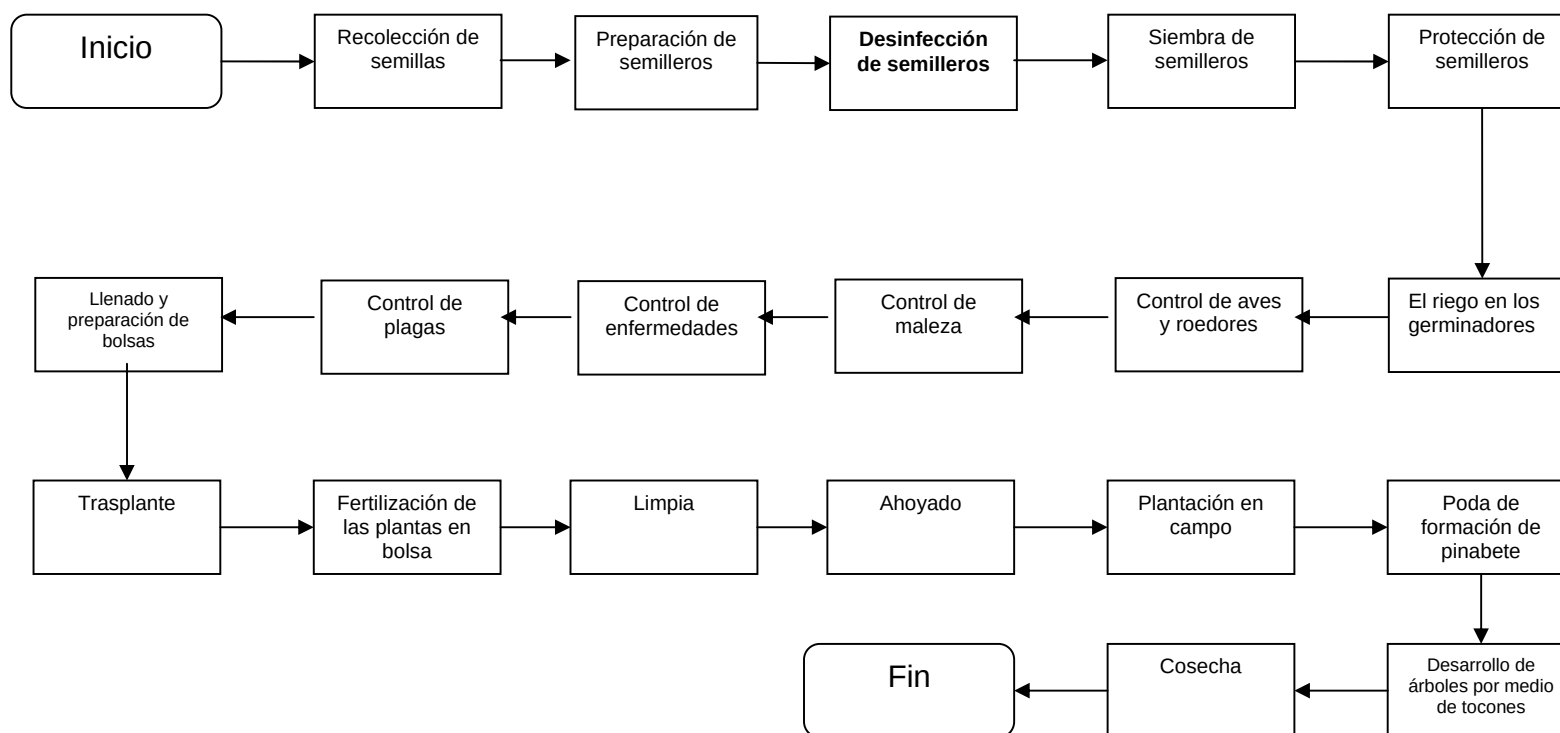
Gráfica 45 Municipio San Juan Ostuncalco, Departamento de Quetzaltenango Proyecto: Producción de Pinabete Flujo del Proceso Productivo, Nivel Tecnológico Nivel II Fincas Sub familiares Año: 2005
