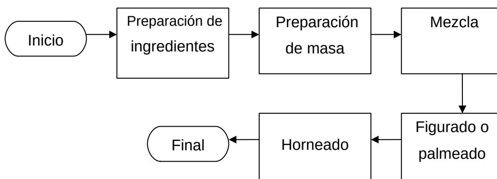
Gráfica 22 Municipio de San Juan Ostuncalco Departamento de Quetzaltenango Flujograma del Proceso Productivo Producción de Pan Dulce y Francés Pequeño Artesano Año: 2005
