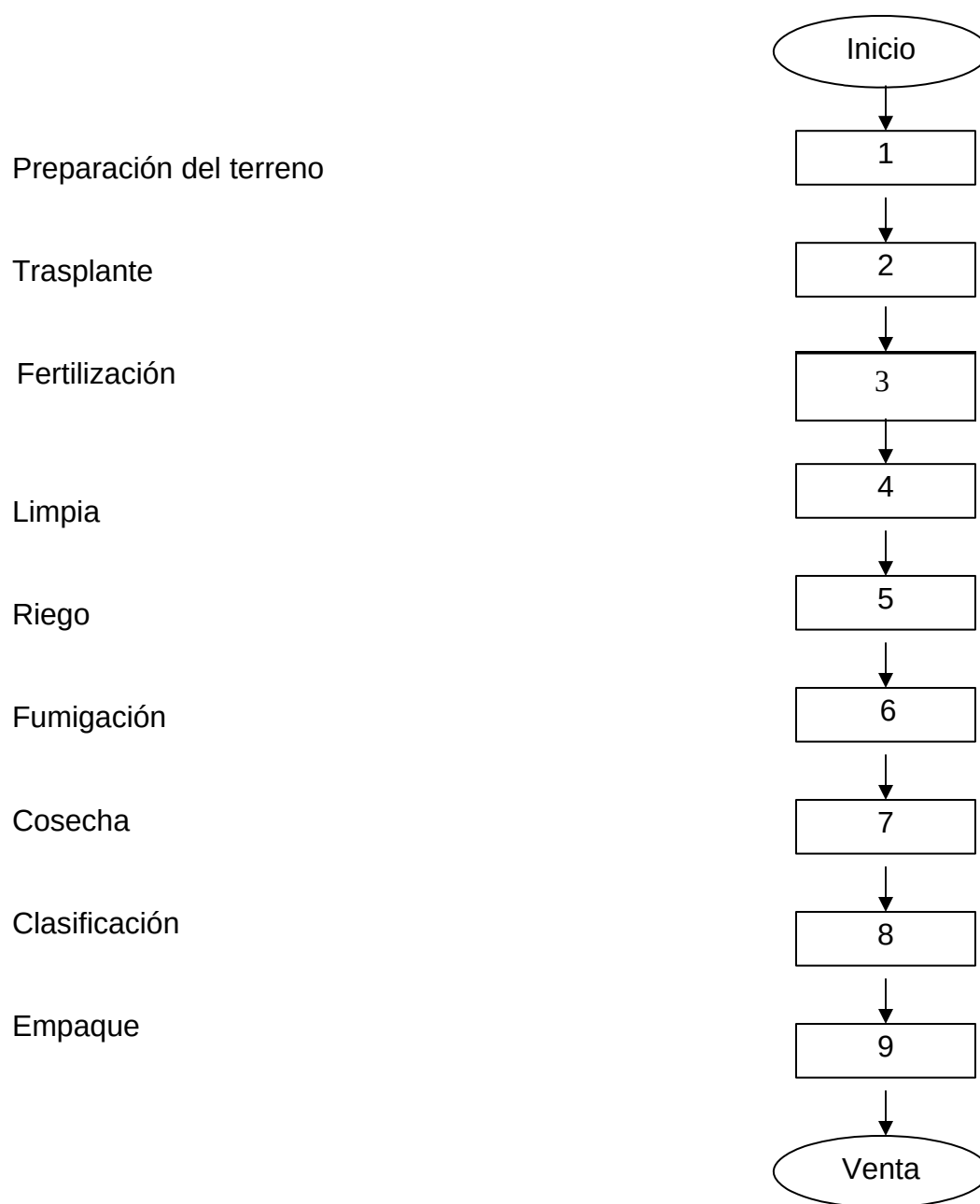
Gráfica 47 Municipio de Flores Costa Cuca - Quetzaltenango Proyecto: Producción de chile pimiento Flujograma del proceso productivo Año: 2005
