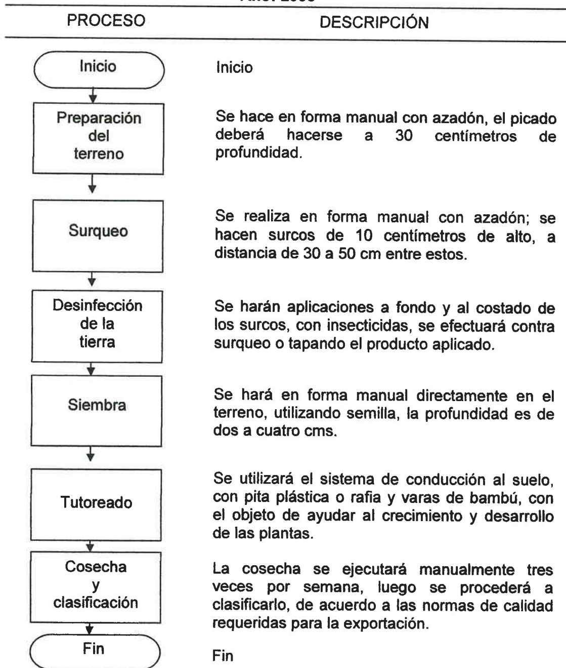
Gráfica 4 Municipio de Cantel – Departamento de Quetzaltenango Proyecto: Producción de ejote francés Flujograma del proceso productivo Año: 2005
