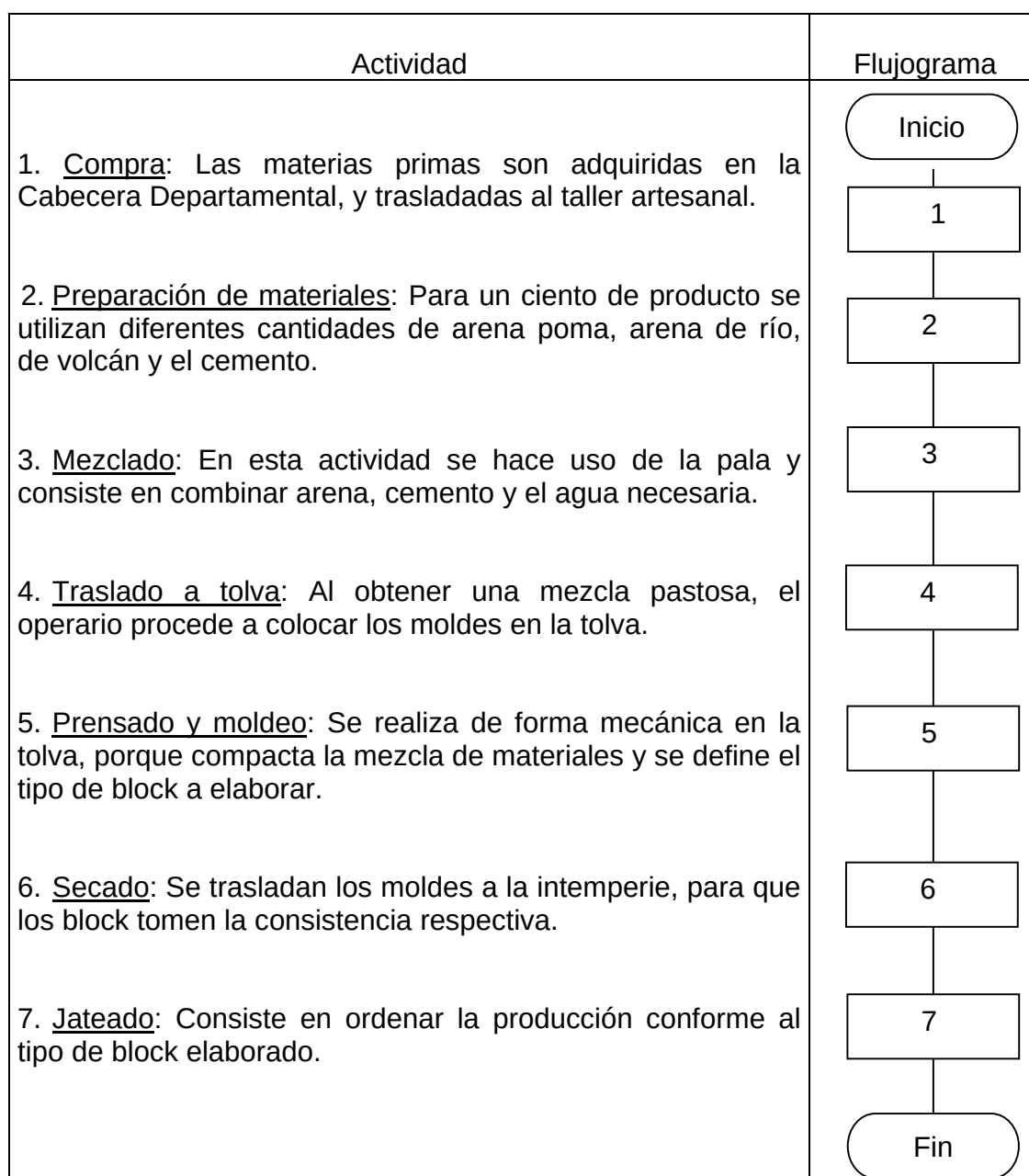
Gráfica 1 Sibilia – Quetzaltenango Elaboración de block Mediano artesano Flujograma del proceso productivo Año 2005
