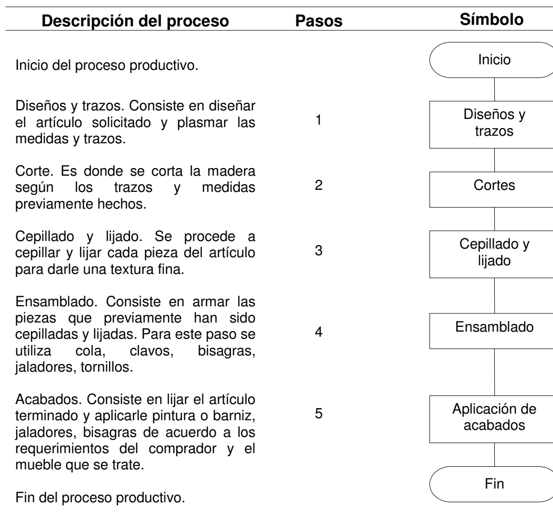
Gráfica 5 Municipio de San José Chacayá - departamento de Sololá Carpintería Pequeño artesano Flujograma del proceso productivo Año 2006
