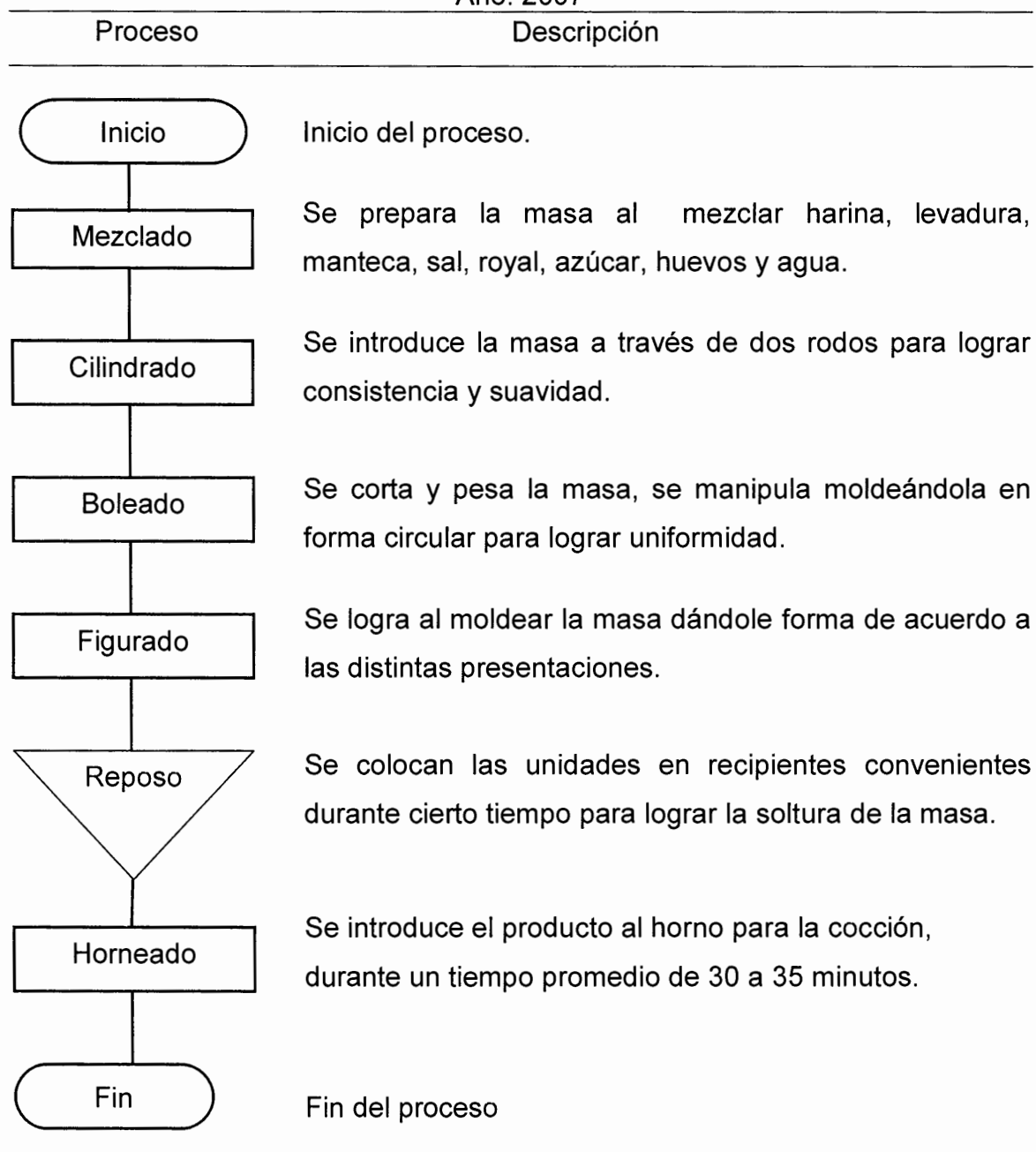
Gráfica 2 Municipio de San Jerónimo – Departamento de Baja Verapaz Pan Francés y Dulce Pequeño Artesano Flujograma del Proceso Productivo Año: 2007
