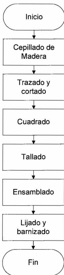
Gráfica 4 Municipio de San Antonio Senahú – Departamento de Alta Verapaz Productos de Carpintería Mediano Artesano Flujograma del Proceso Productivo de un Ropero Año: 2007
