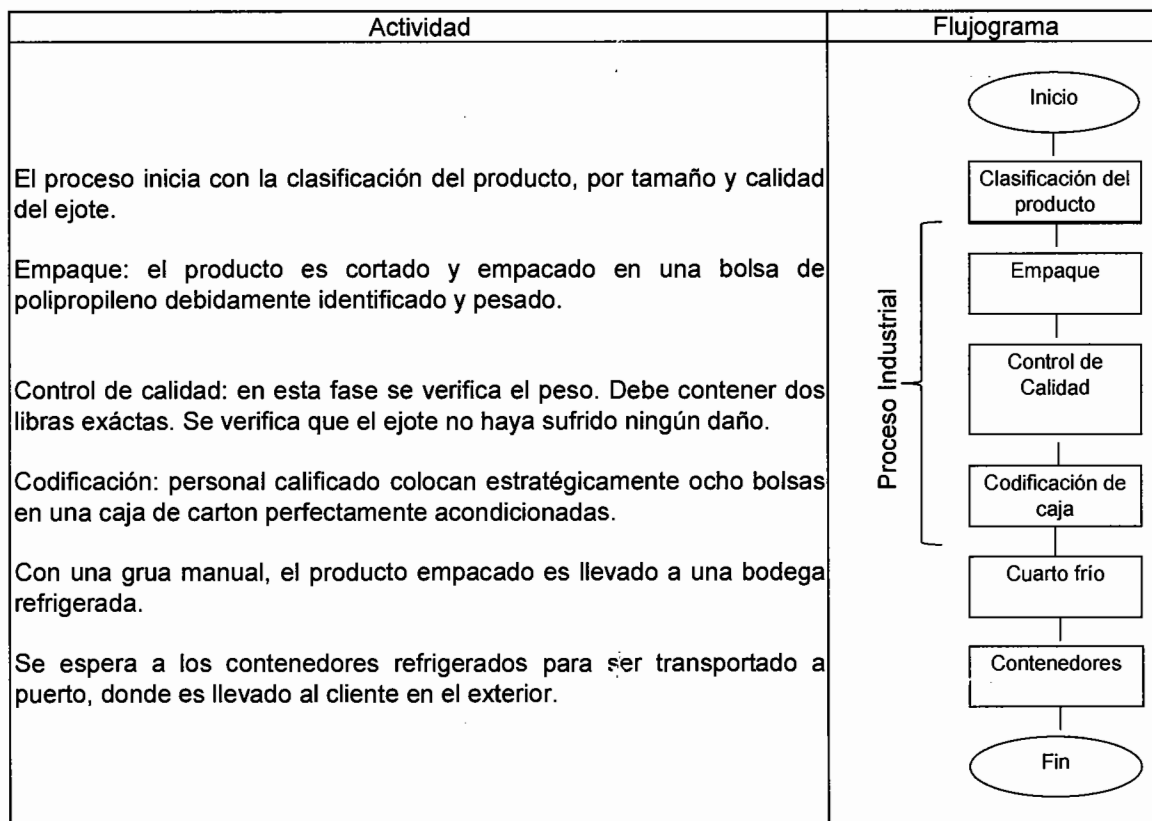
Gráfica 4 Municipio de Uspantán, departamento de Quiché Empacado de Ejote Francés Flujograma del Proceso Productivo Año: 2008
