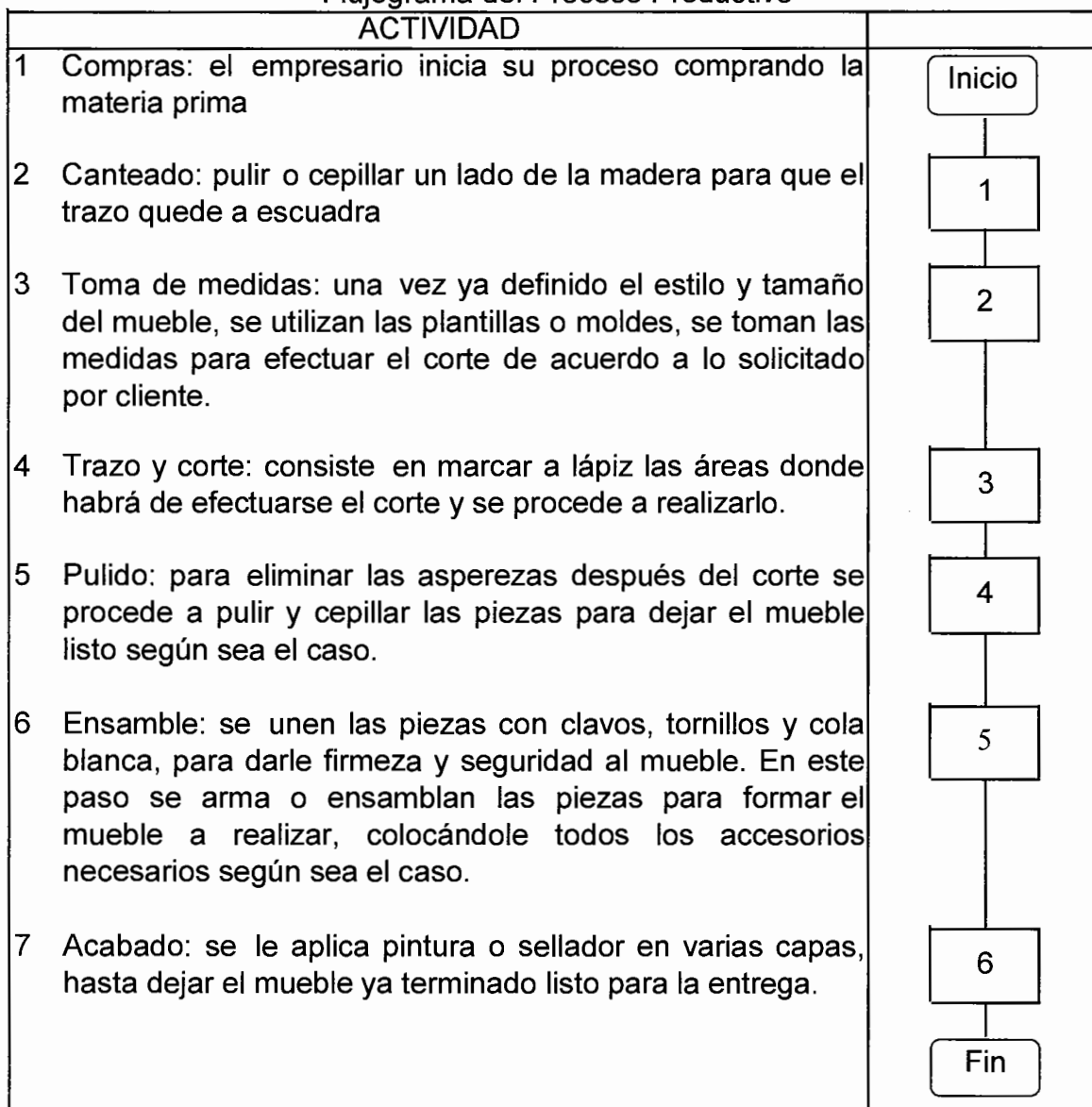
Grafica 2 Municipio de Santa María Nebaj, Departamento de Quiché Carpintería Flujograma del Proceso Productivo
