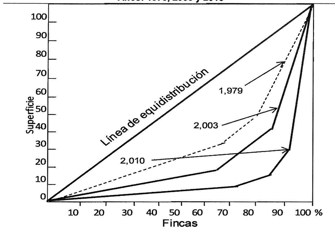
Gráfica 2 Municipio de Malacatán - Departamento de San Marcos Curva de Lorenz Años: 1979, 2003 y 2010
