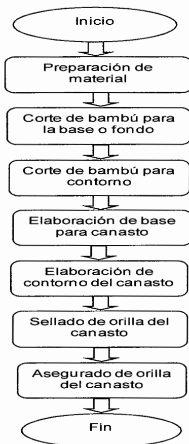
Gráfica 4 Municipio de San Francisco Zapotitlán, departamento de Suchitepéquez Elaboración de canastos de bambú Flujograma del proceso productivo Año: 2010
