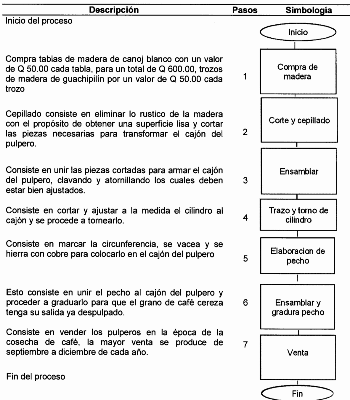
Gráfica 3 Municipio de Santo Tomás La Unión - Suchitepéquez Elaboración de Pulperos Flujograma del Proceso de Elaboración Año: 2010
