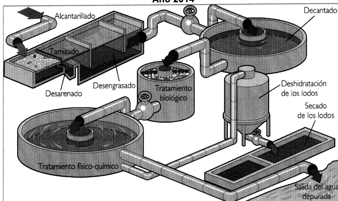
Imagen 1 Municipio de Teculután, departamento de Zacapa Esquema Gráfico de Planta de Tratamiento Año 2014
