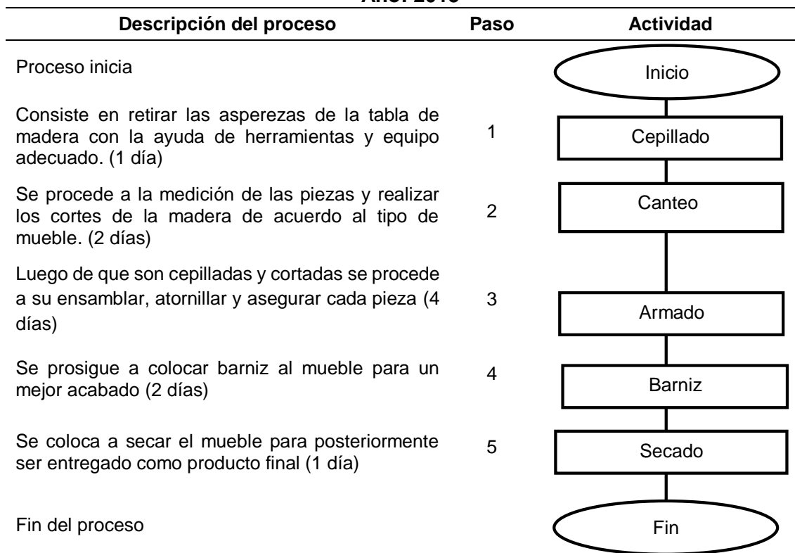
Gráfica 3 Municipio de San Antonio Suchitepéquez, departamento de Suchitepéquez Flujograma del proceso productivo Carpintería Año: 2015
