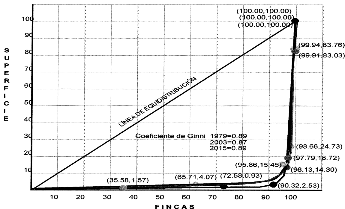
Gráfica 1 Municipio de Nuevo San Carlos, departamento de Retalhuleu Curva de Lorenz Año: 1979, 2003 y 2015
