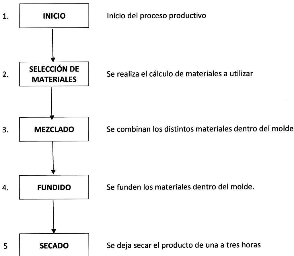
Gráfica 2 Municipio de La Democracia, Departamento de Huehuetenango Flujograma del Proceso Productivo de Elaboración de Productos de Cemento Año: 2016
