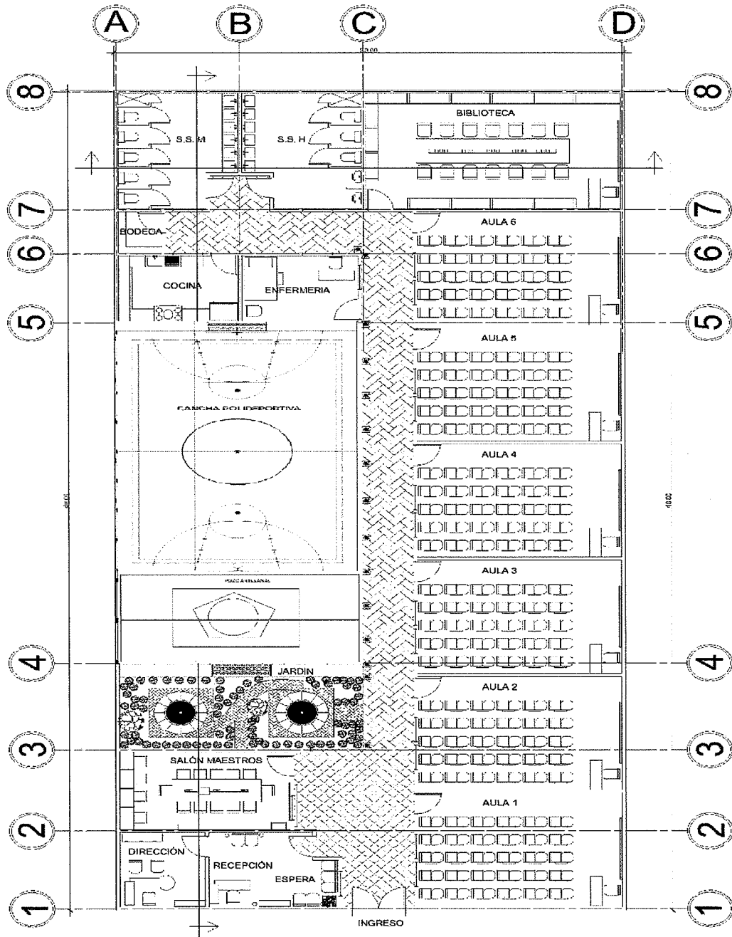
PLANTA ARQUITECTÓNICA INSTITUTO DIVERSIFICADO LA DEMOCRACIA, SAN MARCOS ESCALA 1/100
