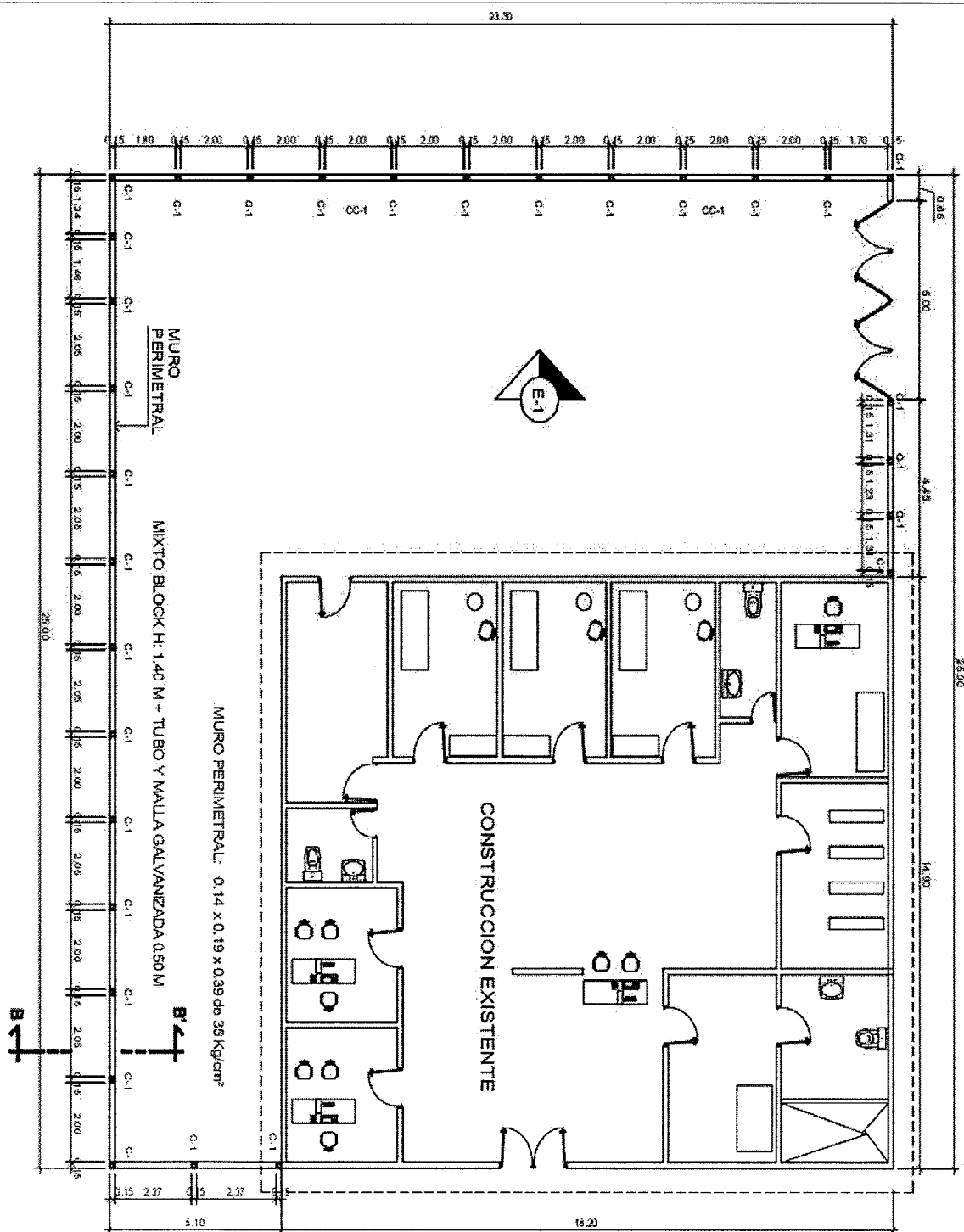
Imagen 1 Aldea Santa Clara, municipio La Reforma, departamento de San Marcos Croquis de mejoramiento puesto de salud Año 2018
