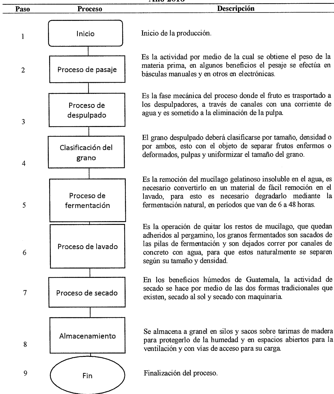
Gráfica 4 Aldea La Conquista, caserío San José Paríán y cantón Barrios, Municipio de Nuevo Progreso, Departamento de San Marcos Producción agroindustrial Flujograma del proceso de producción Año 2018
