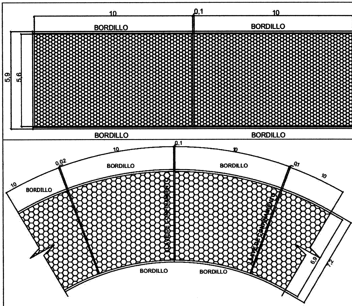
Imagen 2 Municipio de Santa María Visitación, departamento de Sololá Proyecto: Mejoramiento camino, caserío Chuipoj Plano planta de adoquinamiento de la calle Año: 2017
