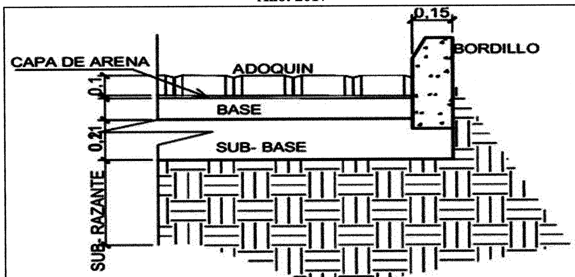
Imagen 1 Municipio de Santa María Visitación, departamento de Sololá Proyecto: Mejoramiento camino, caserío Chuipoj Plano colocación de base, sub-base y adoquín Año: 2017
