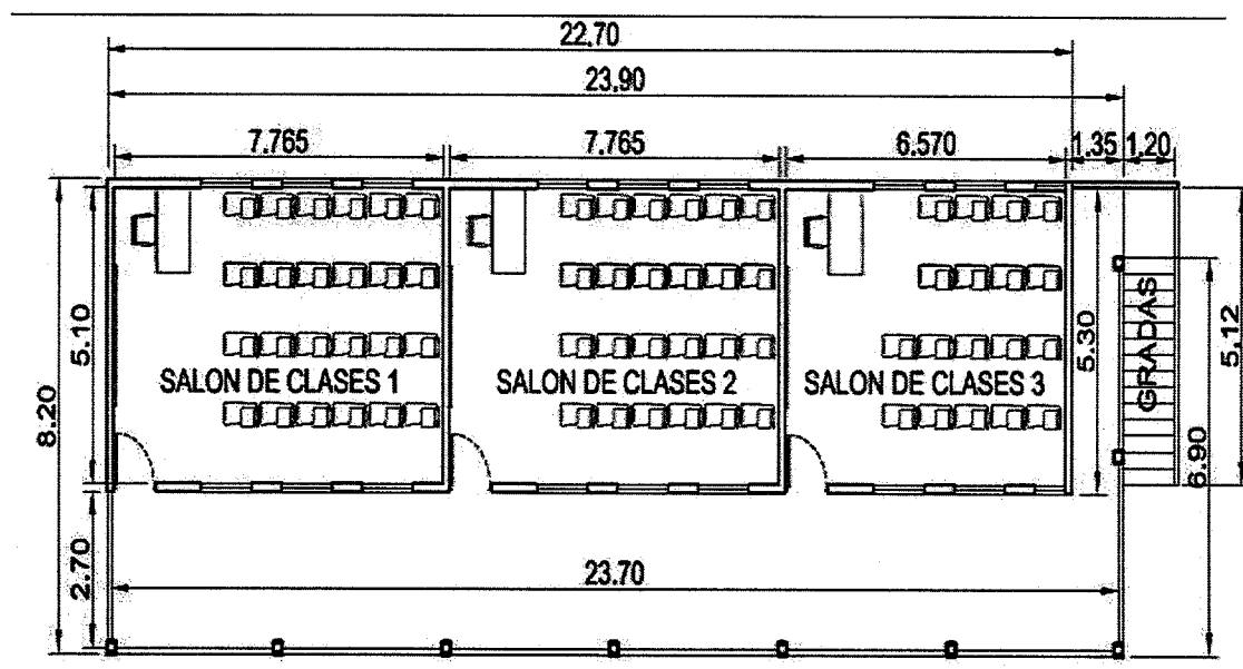
Figura 3 Aldea El Limón Municipio de Santa Catarina Mita, departamento de Jutiapa Proyecto: ampliación de escuela oficial rural mixta Diseño planta de segundo nivel Año: 2019
