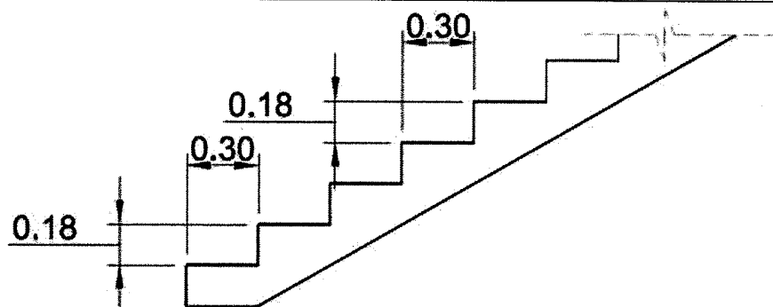
Figura 4 Aldea El Limón Municipio de Santa Catarina Mita, departamento de Jutiapa Proyecto: ampliación de escuela oficial rural mixta Diseño planta de gradas Año: 2019
