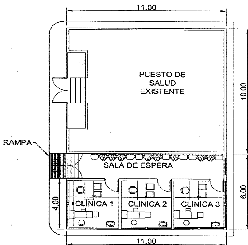
Figura 2 Aldea El Limón Municipio de Santa Catarina Mita, departamento de Jutiapa Proyecto: ampliación del puesto de salud Plano de ampliación Año: 2019
