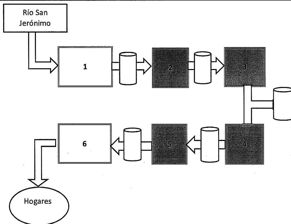
Gráfica 4 Aldea Los Jocotes, municipio de San Jerónimo, departamento de Baja Verapaz Diagrama de funcionamiento, Planta de tratamiento de agua Potable Año: 2020
