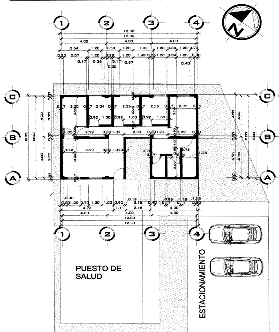
Imagen 6 Aldeas Canoas Altas y Canoas Bajas, municipio de San Andrés Semetabaj, departamento de Sololá Proyecto: Construcción Centro de Psicología, Aldea Canoas Bajas Planta arquitectónica acotada Año: 2017
