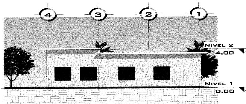
ELEVACIÓN - NORTE
