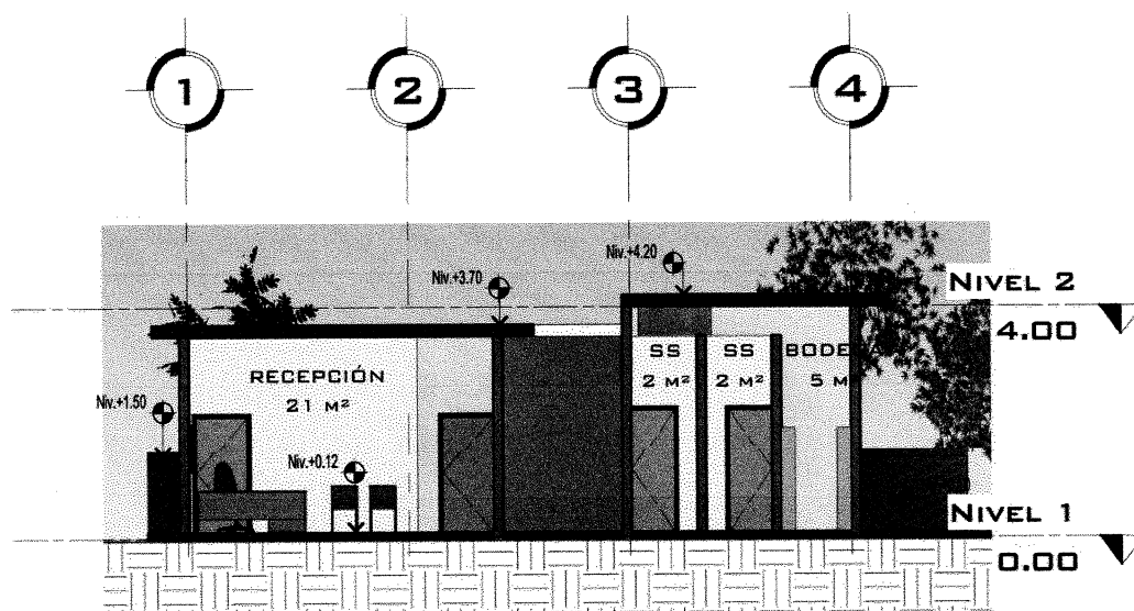
Imagen 5 Aldeas Canoas Altas y Canoas Bajas, municipio de San Andrés Semetabaj, departamento de Sololá Proyecto: Construcción Centro de Psicología, Aldea Canoas Bajas Sección A y B Año: 2017
