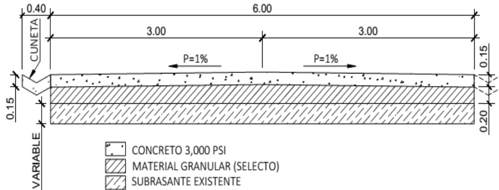
SECCIÓN TRANSVERSAL TÍPICA DE CALLE
