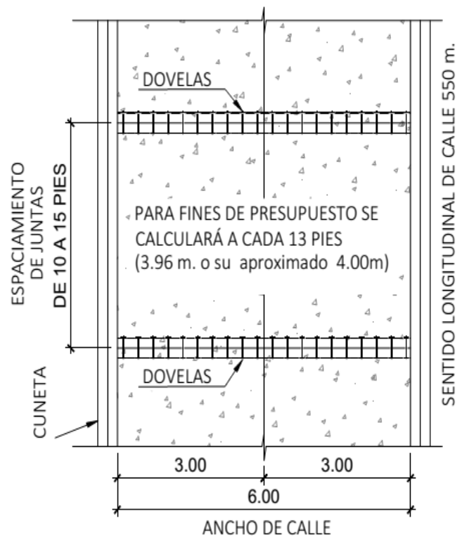
PLANTA TÍPICA DE CALLE
