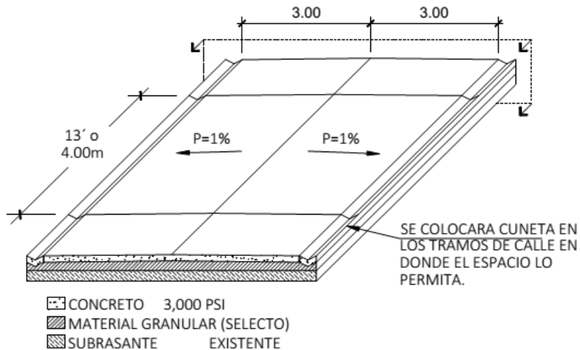
PERSPECTIVA JUNTAS DE CALLE
