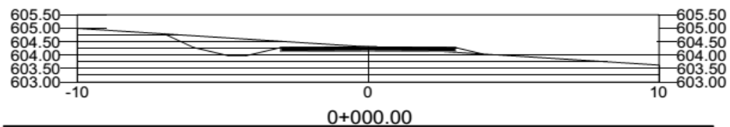
DETALLE TÍPICO SOBRE CORTE Y RELLENO DE CALLE
