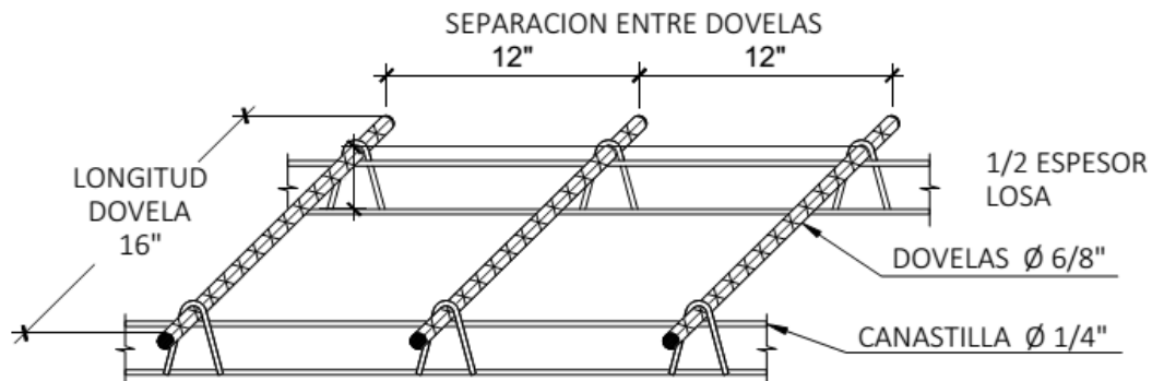
DETALLE CANASTILLA PARA DOVELAS
