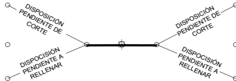
DETALLE TÍPICO SOBRE CORTE Y RELLENO DE CALLE
