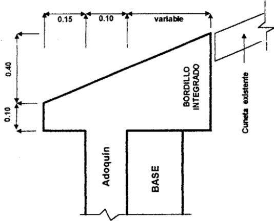
DETALLE BORDILLO - CUNETETA
