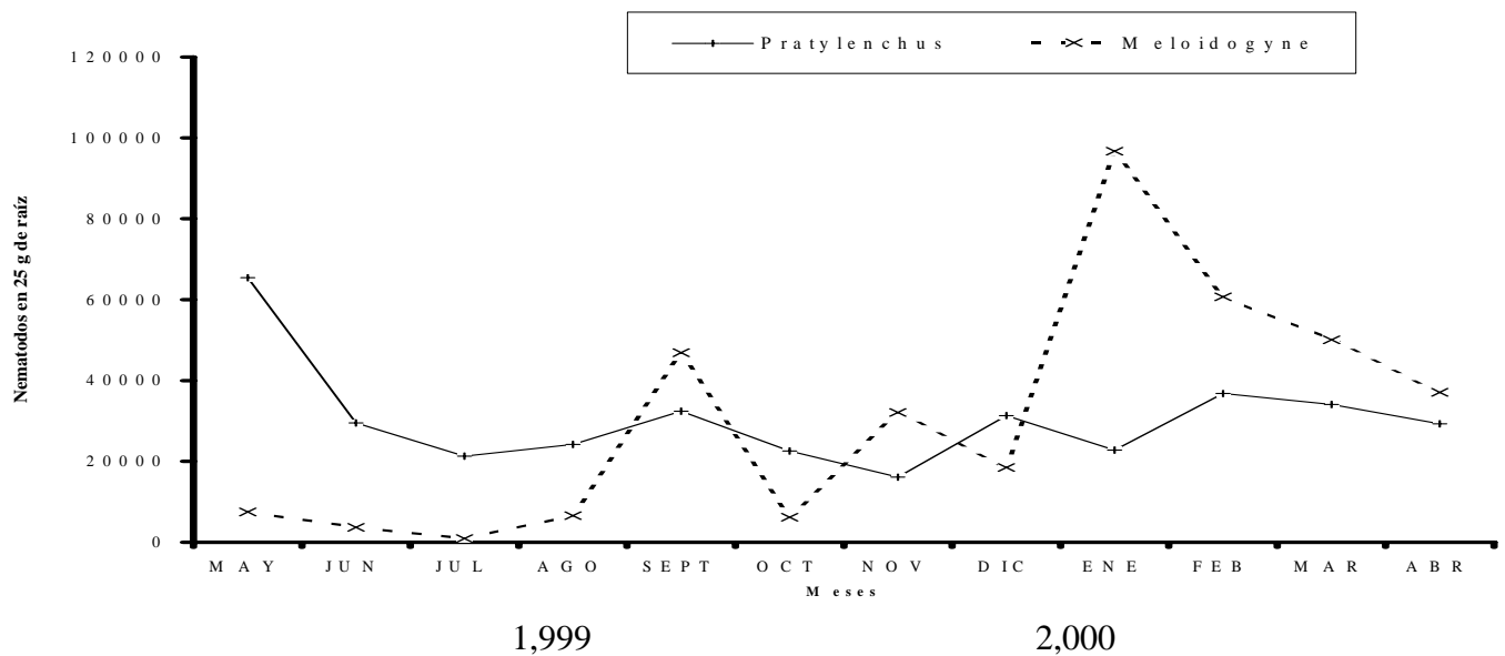
Figura 3. Variación estacional del Pratylenchus y Meloidogyne en la finca Unión Tacaná, Nuevo Progreso, San Marcos. Ciclo 1,999-2,000.
