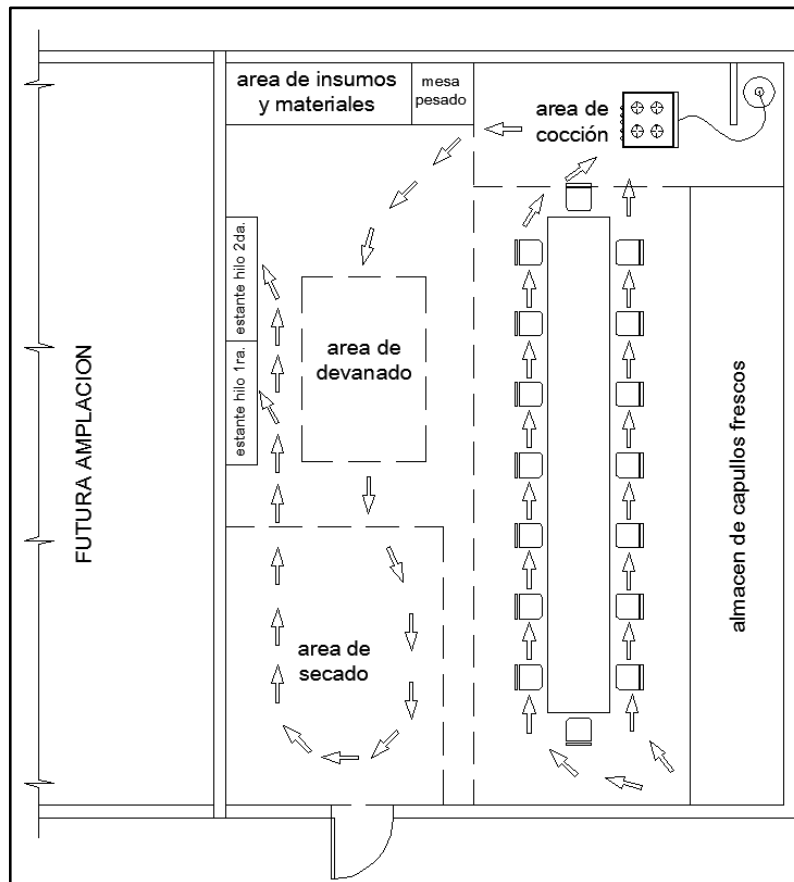
Figura 9. Distribución de áreas de trabajo
