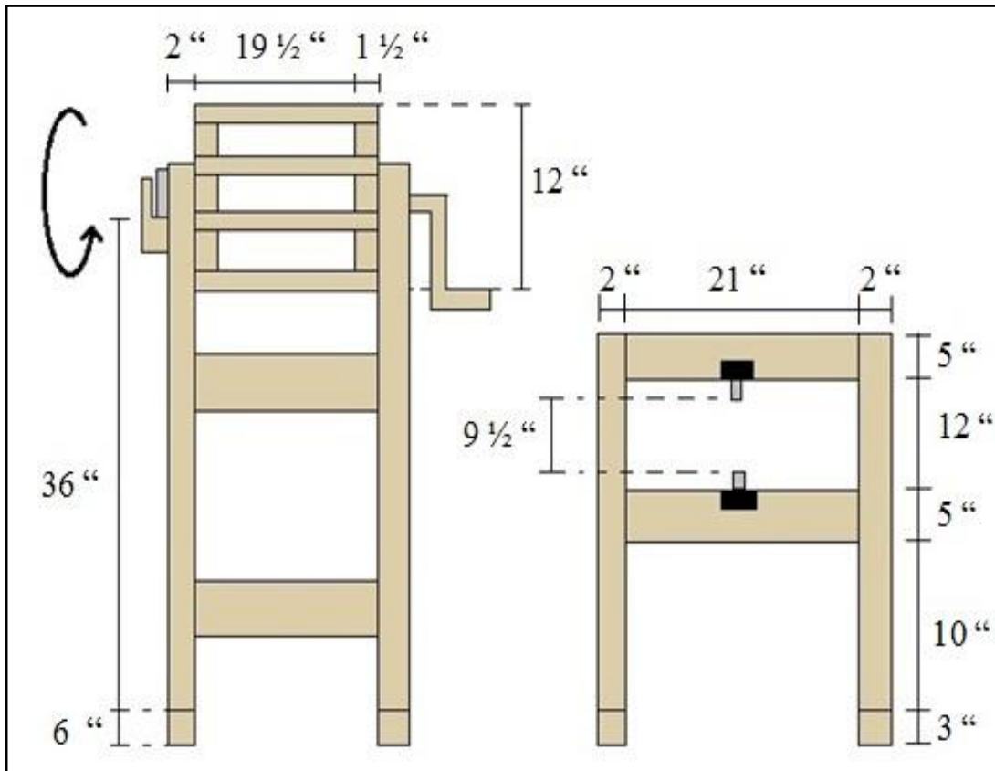
Figura 16. Vista frontal devanadora artesanal
