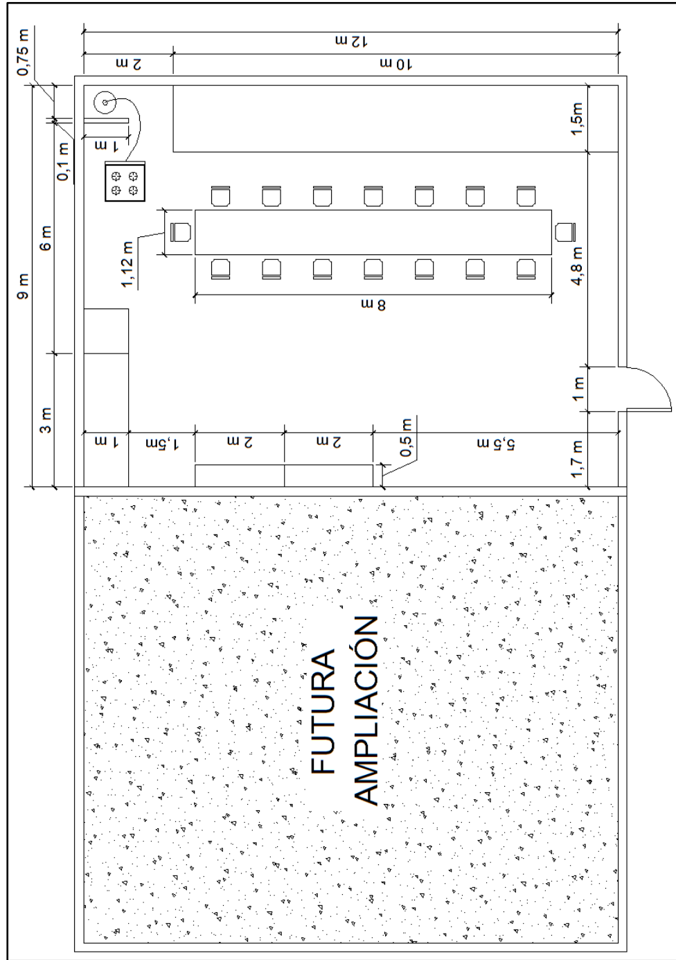
Figura 7. Distribución de planta, 2da etapa
