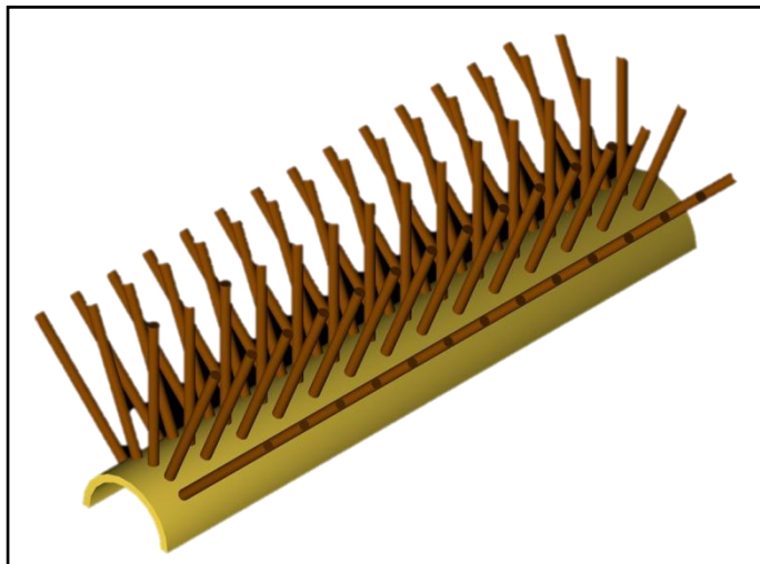
Figura 12. Vista isométrica de encapullador tipo rodalina
