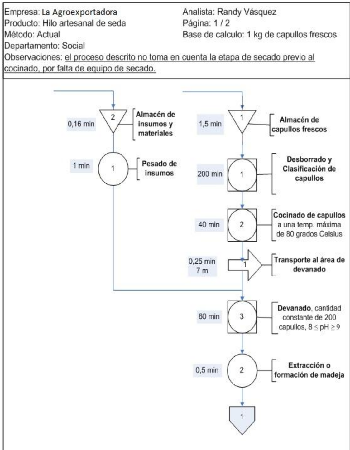
Figura 8. Diagrama de flujo producción de hilo de seda
