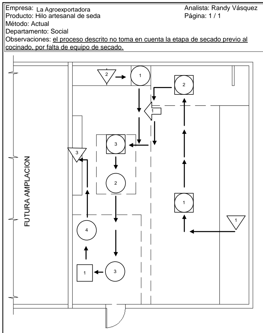
Figura 10. Diagrama de recorrido, producción artesanal de seda
