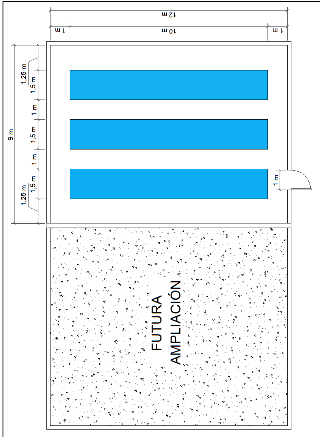
Figura 6. Distribución de planta, primera etapa
