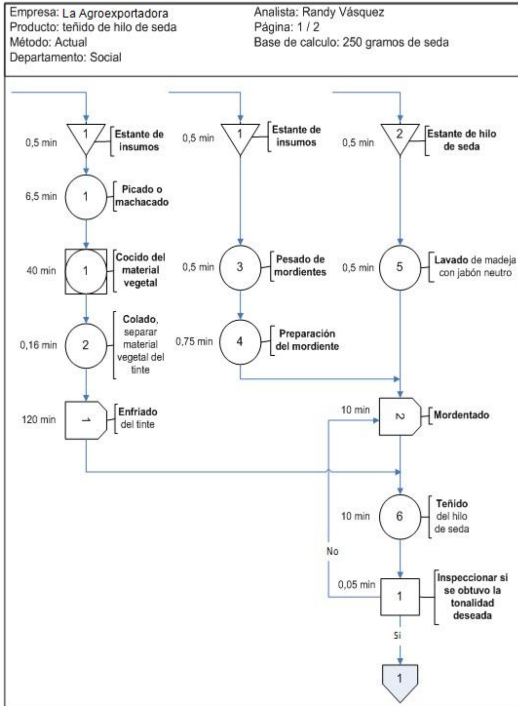
Figura 19. Diagrama de flujo de teñido artesanal
