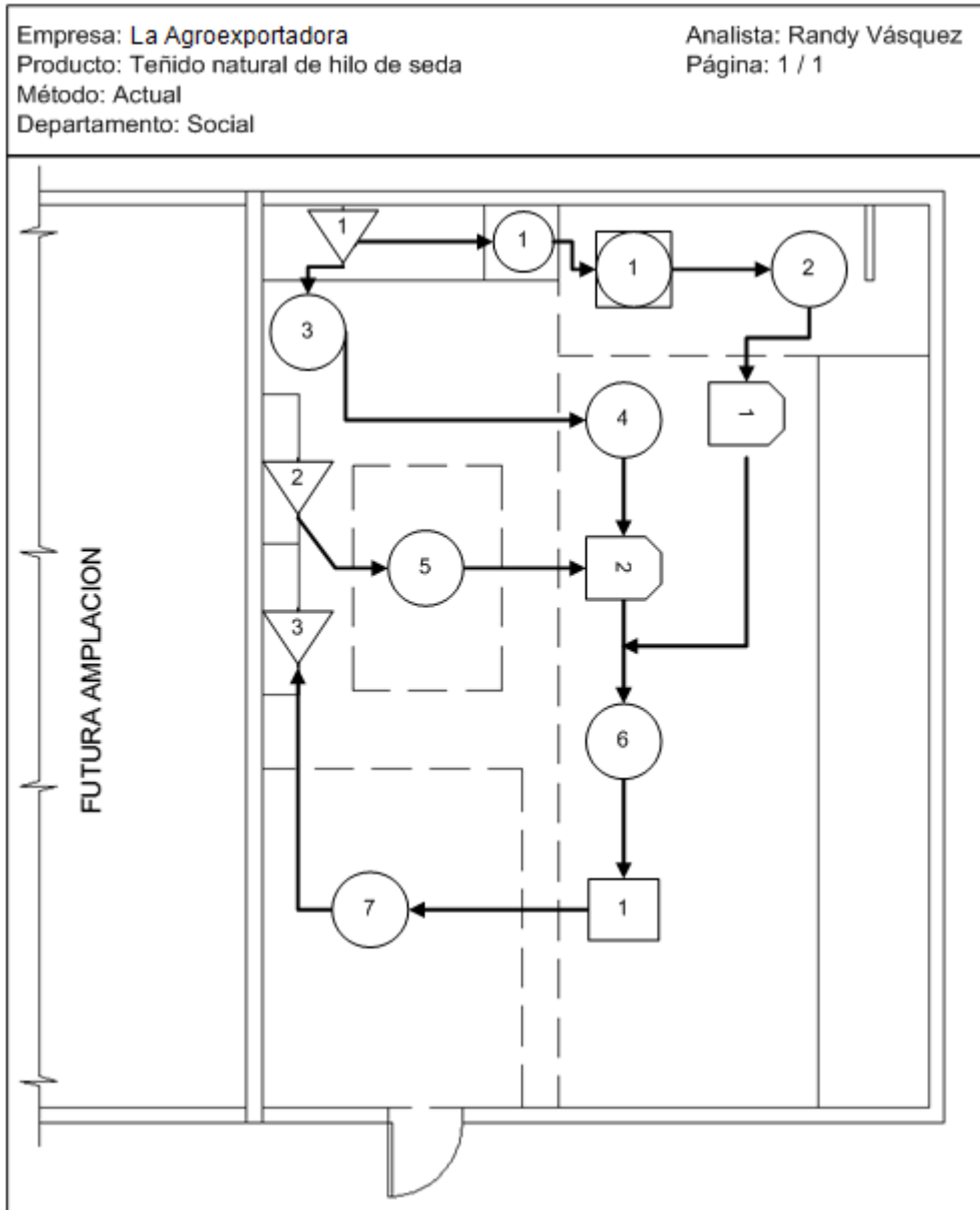
Figura 20. Diagrama de recorrido teñido de seda
