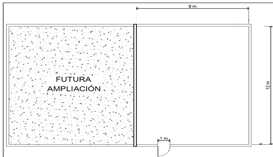
Figura 4. Terreno para la construcción de la planta piloto
