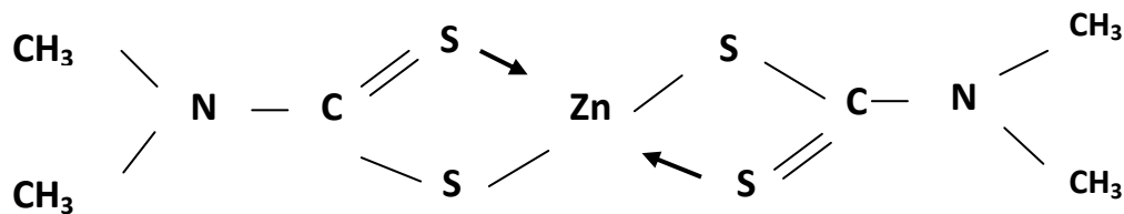
Figura 1. Estructura química de dimetildiocarbamatos
