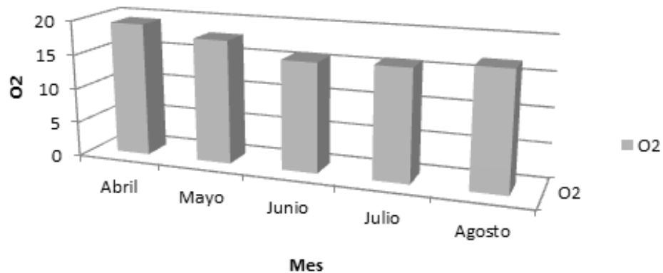
Figura 11. Concentración de O 2
