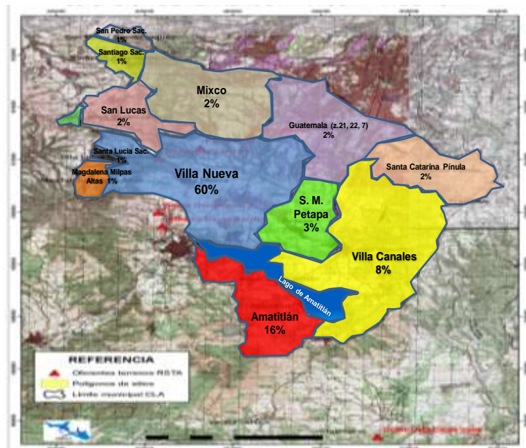
Figura 6. Porcentaje de disposición de desechos sólidos por municipio en el relleno sanitario
