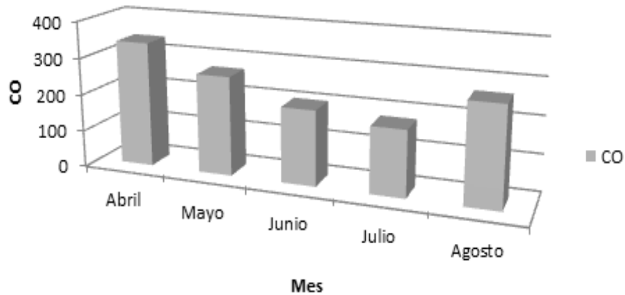
Figura 12. Concentración de CO
