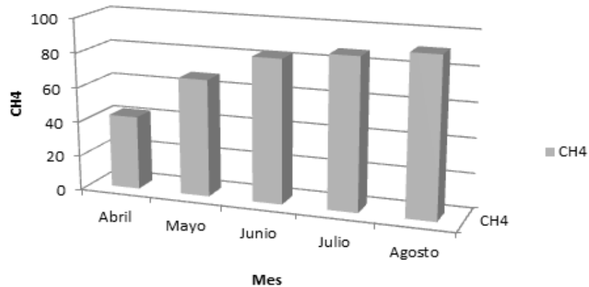
Figura 10. Concentración de CH 4
