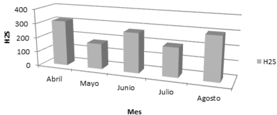
Figura 13. Concentración de H 2 S
