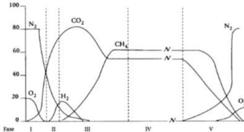
Figura 2. Composición óptima de biogás en una celda de relleno sanitario
