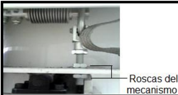
Imagen No. 6. Mecanismo que ayuda a la vibración de la báscula
