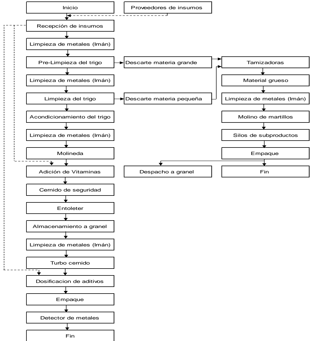
Figura 5. Diagrama de bloques
