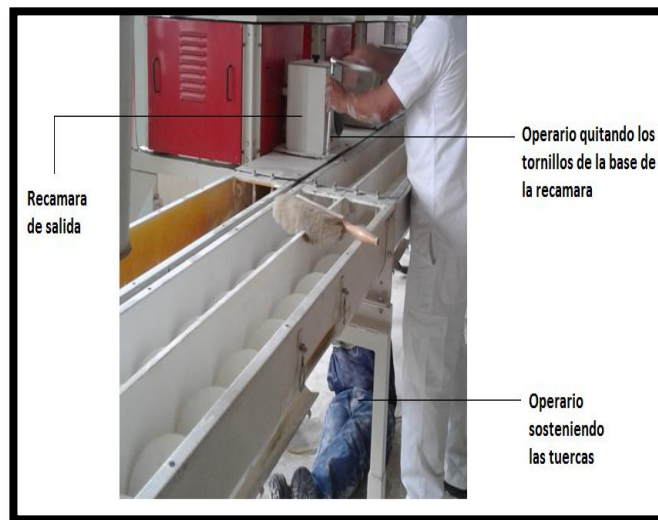
Imagen No.3. Desmontaje de la recámara de salida
