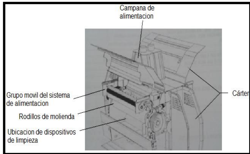
Imagen No. 10. Dibujo didáctico de cómo se observara el banco de molienda totalmente abierto
