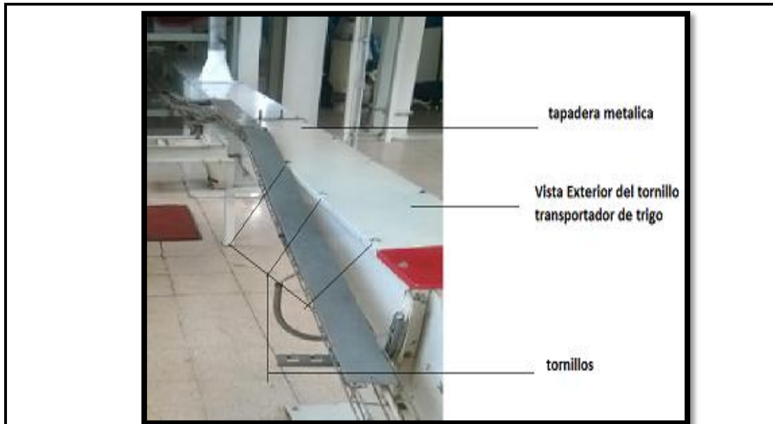
Imagen No. 2. Ubicación de los tornillos a desatornillar.
