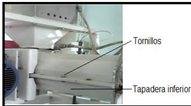
Imagen 4. Ubicación de la tapadera inferior a retirar y los tornillos a desatornillar
