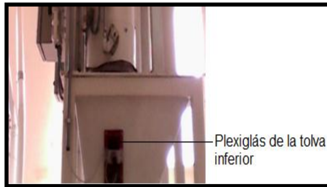
Imagen No. 7. Ubicación de los tornillos a quitar y retirar el plexiglás junto con el sensor.
