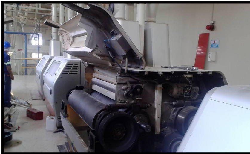
Imagen No. 16. Interior de la tolva de recogida
