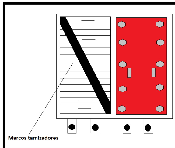
Imagen No. 3. Vista de los marcos ubicados en la recámara de los cernedores
