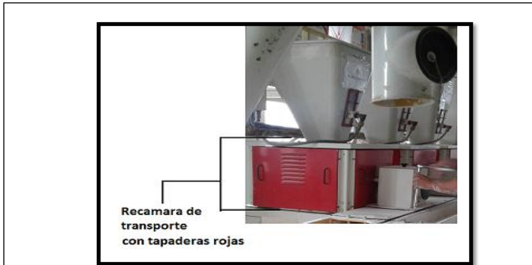
Imagen No.6. Vista exterior de la recámara de transporte con tapaderas de recubrimiento.
