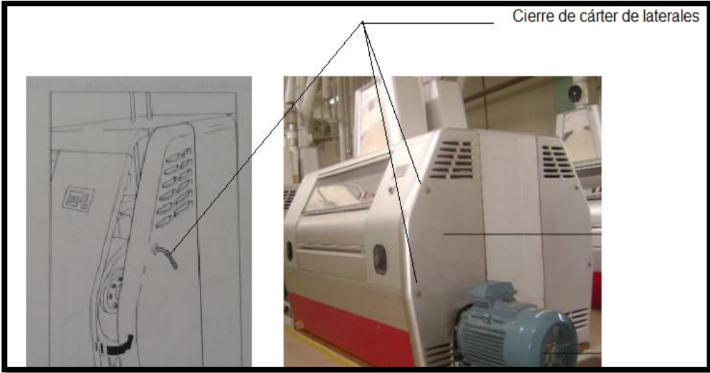
Imagen No. 6. Cierres de carter laterales
