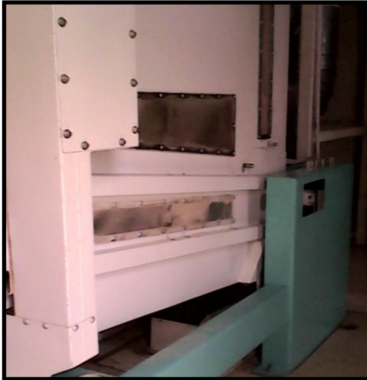
Imagen No. 1. Vista de la zaranda multicleaner ubicada en el cuarto nivel
