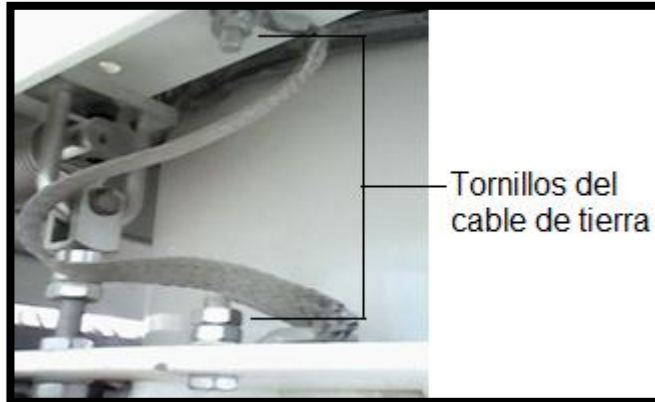
Imagen No. 5. Alambre de tierra a retirar.
