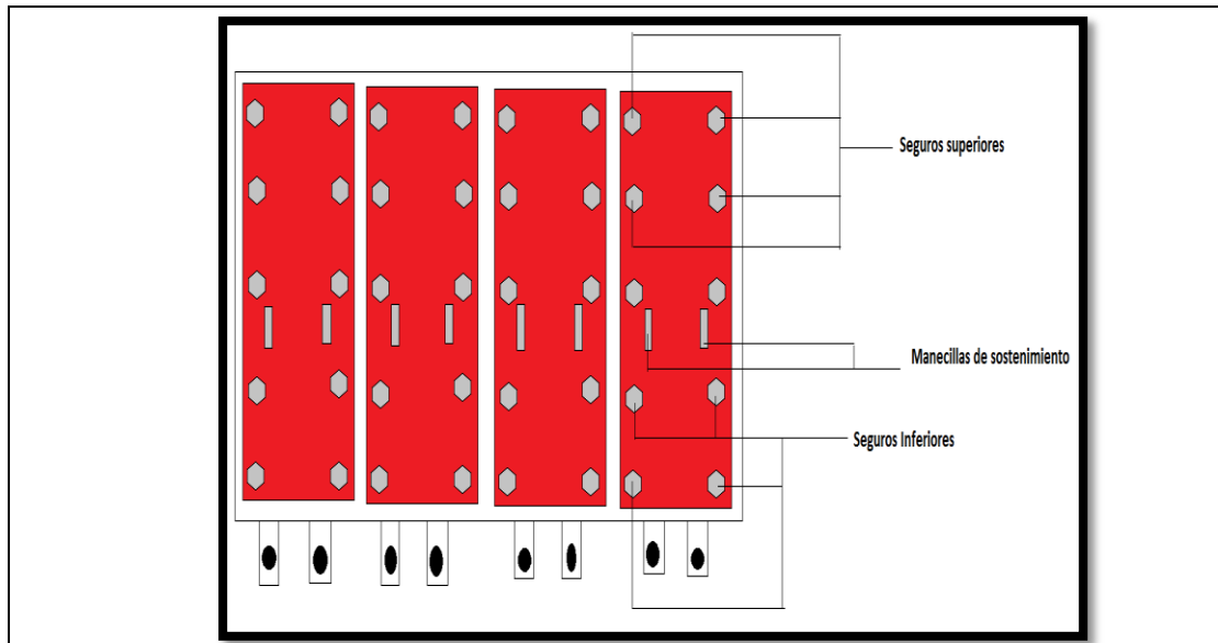
Imagen No. 2. Ubicación de los seguros superiores e inferiores (tornillos hexagonales) y manecillas de las puertas de los cernedores.
