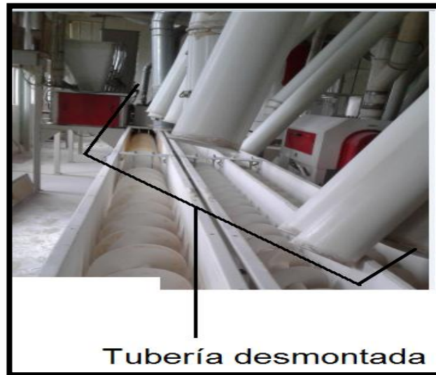
Imagen No. 4. Tubería desmontada lista para ser limpiada y sanitizada
