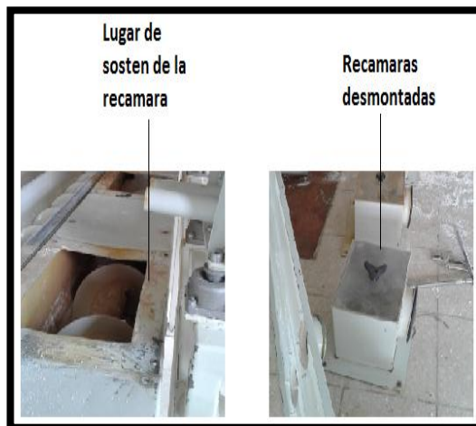
Imagen No. 4. Se observan las recámaras de salida desmontadas.
