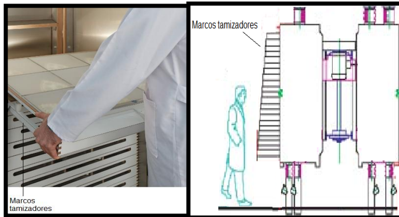
Imagen No. 3. Vista de cómo sacar los marcos ubicados en la recámara de los cernedores
