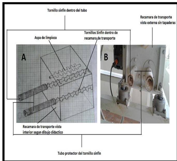
Imagen No. 7. A) se observa el dibujo didáctico de cómo quedará la recámara de transporte interiormente esta cuenta con dos tornillos sinfín y un aspa de limpieza. B) imagen exterior de cómo se observan los tubos que cubren los tornillos sinfín.
