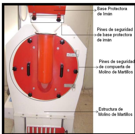
Imagen No. 1. Vista y partes del molino de martillos
