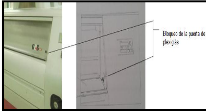
Imagen No. 4. Bloqueo de la puerta de plexiglás
