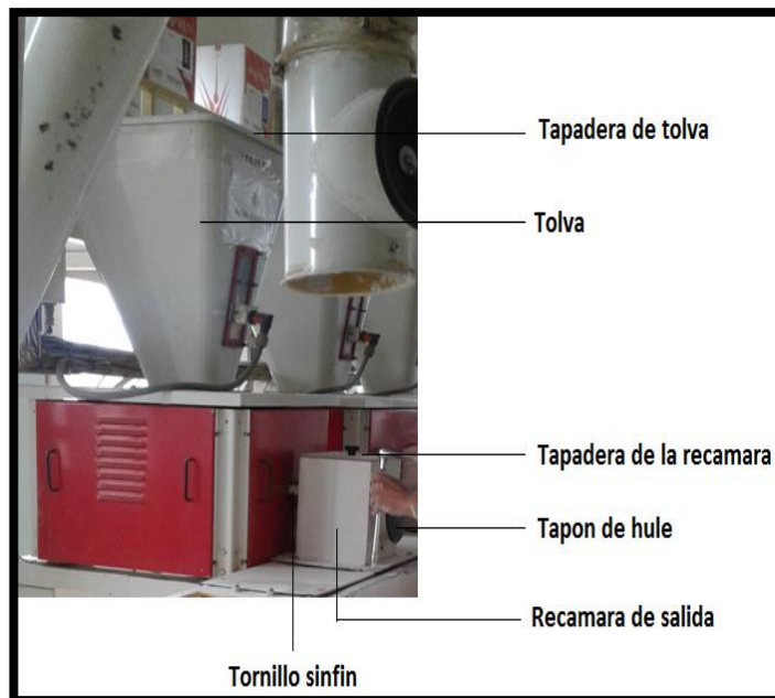
Imagen No. 1. Vista del equipo de dosificación de vitaminas para la harina de trigo
