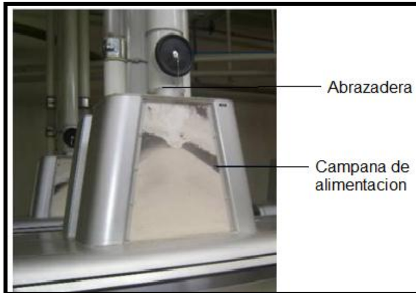
Imagen No. 3. Partes a desmontar de la campana de alimentación
