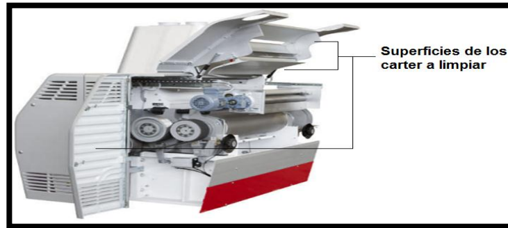
Imagen No. 14. Superficies de los carter a limpiar
