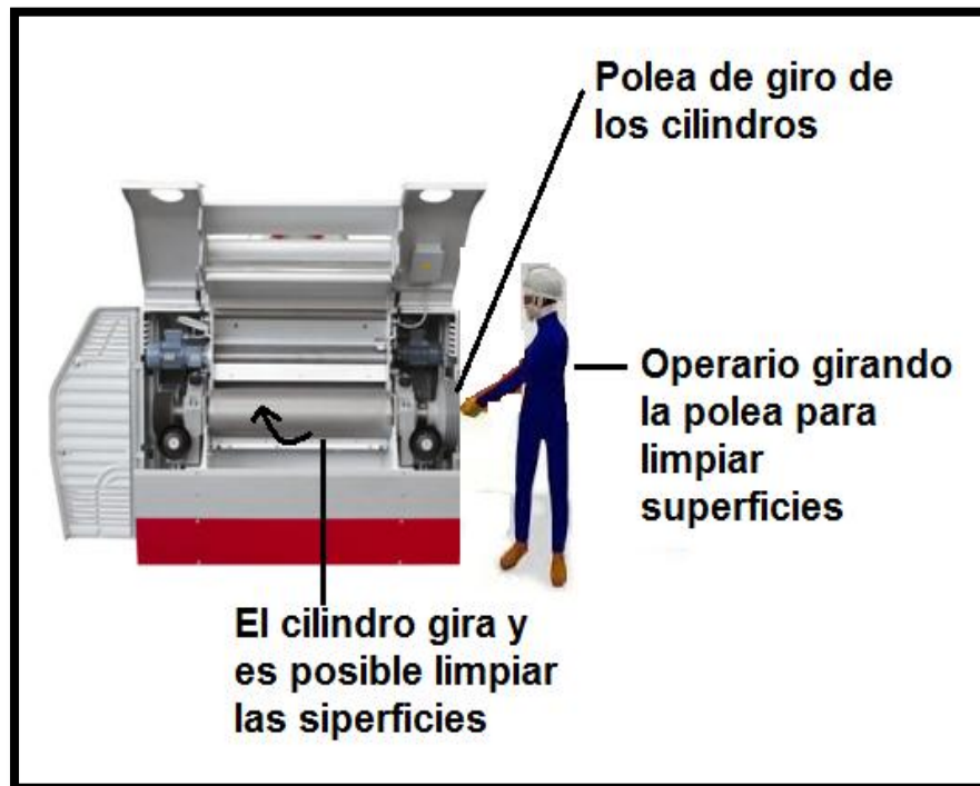
Imagen No. 14. Forma de limpieza de los cilindros
