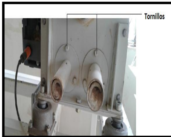
Imagen No. 8. En la imagen se observan los tornillos a quitar
