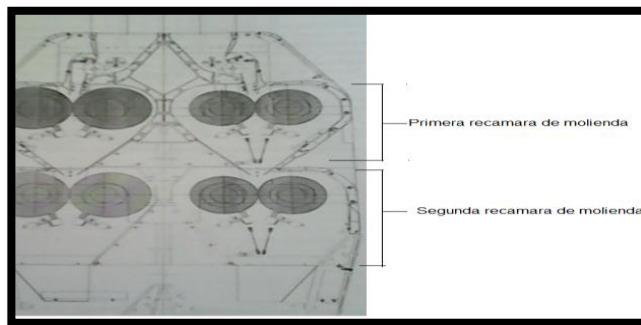
Imagen No. 2. Esquema interno lateral de los 8 cilindros de molienda.
