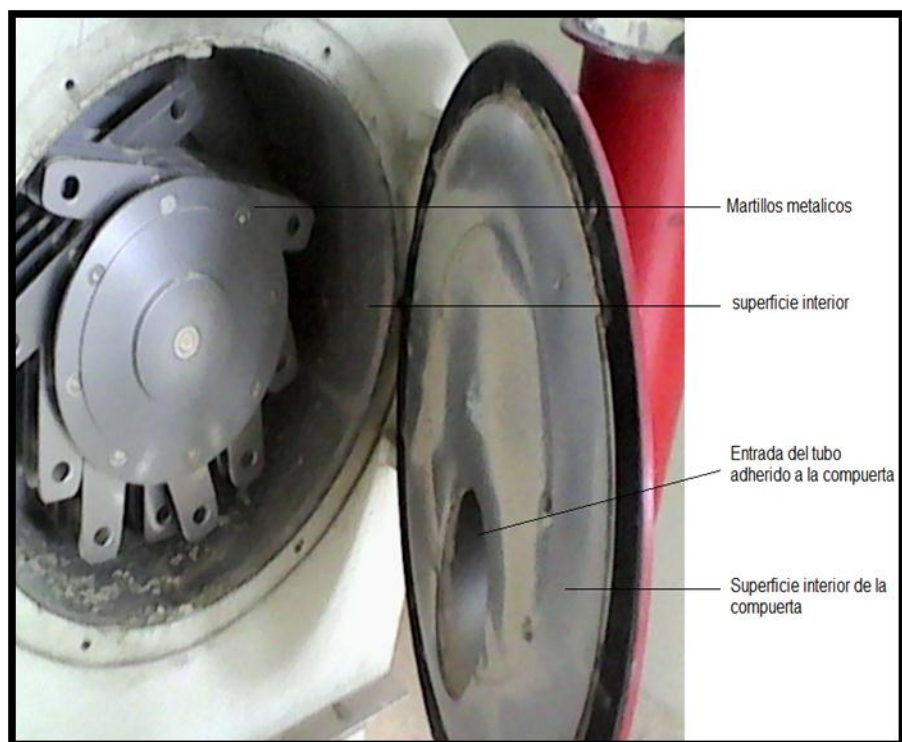
Imagen No. 4. Descripción de las superficies a limpiar
