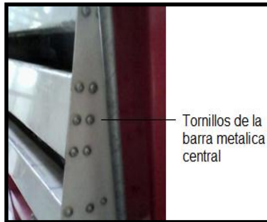
Figura. 4. Se observan los seis tornillos a quitar estos se encuentra en ambos lados laterales.
