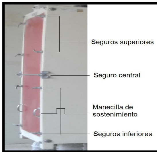
Imagen No. 2. Ubicación de los seguros y manecillas de las puertas del cernedor.
