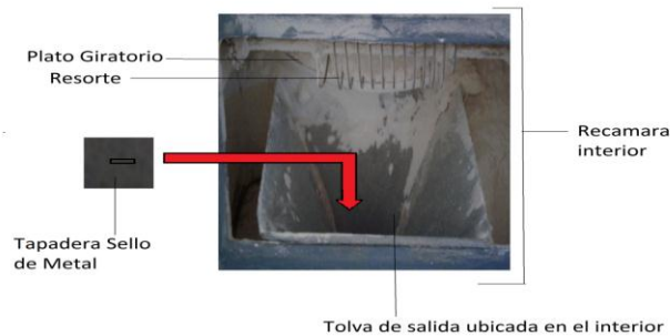
Imagen No. 4. La flecha indica donde se coloca la tapadera sello de metal para evitar caídas de residuos al tornillo transportador.
