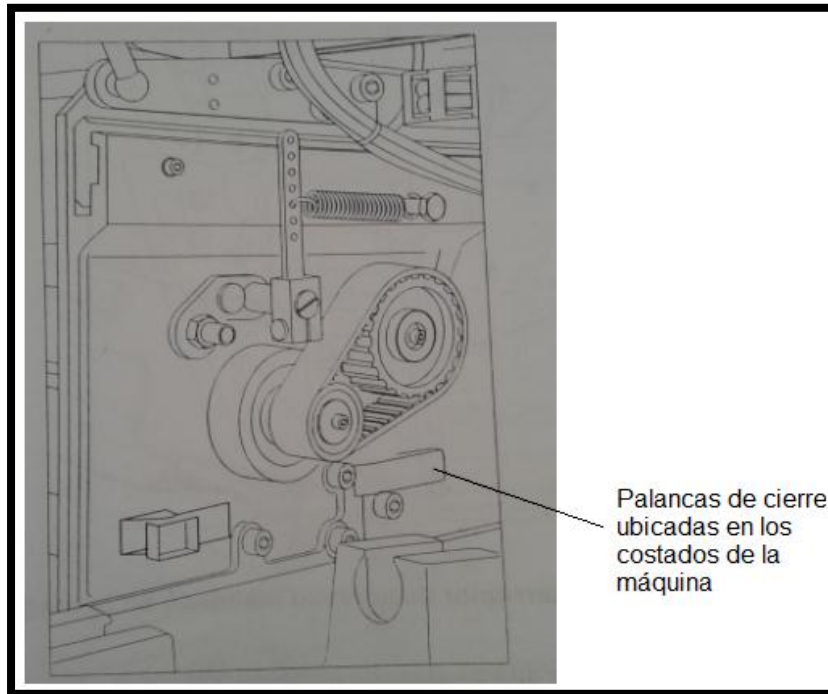
Imagen No. 10. Observación de las palancas de cierre ubicadas en los costados de la máquina
