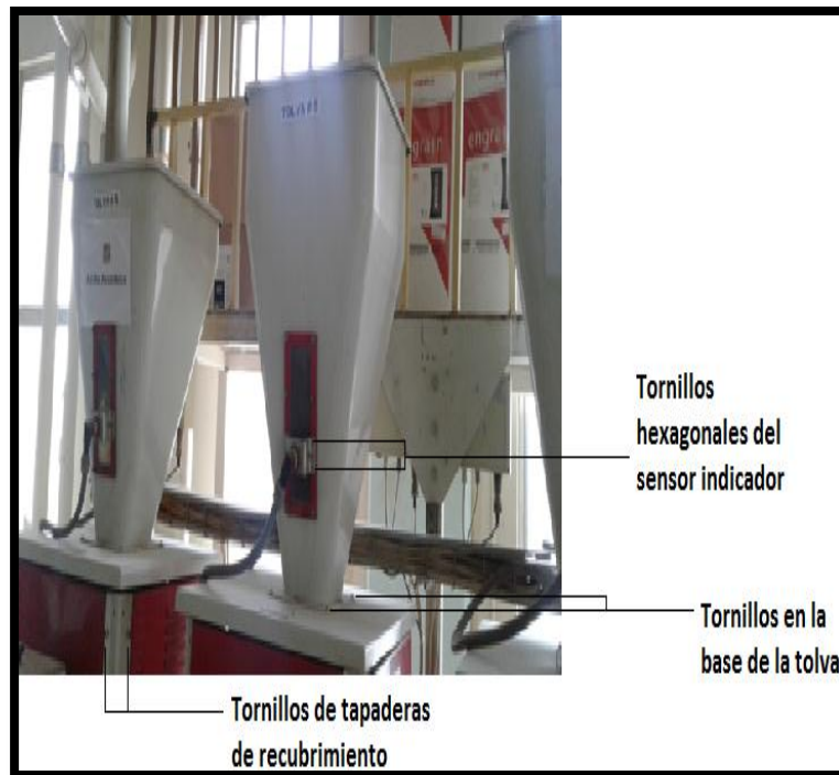
Imagen No. 5. Tornillos a quitar para el desmontaje y montaje para la limpieza y sanitización
