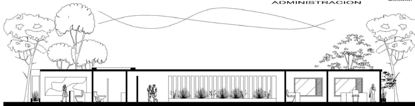
CORTE ADMINISTRACION Escala: 1/ 100
