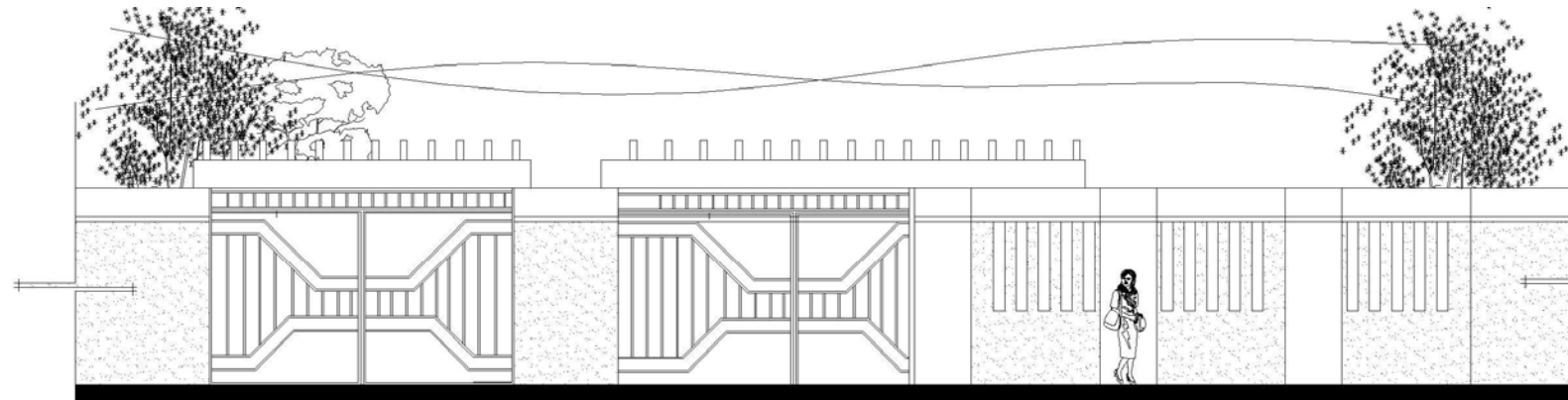
• ELEVACION 1
