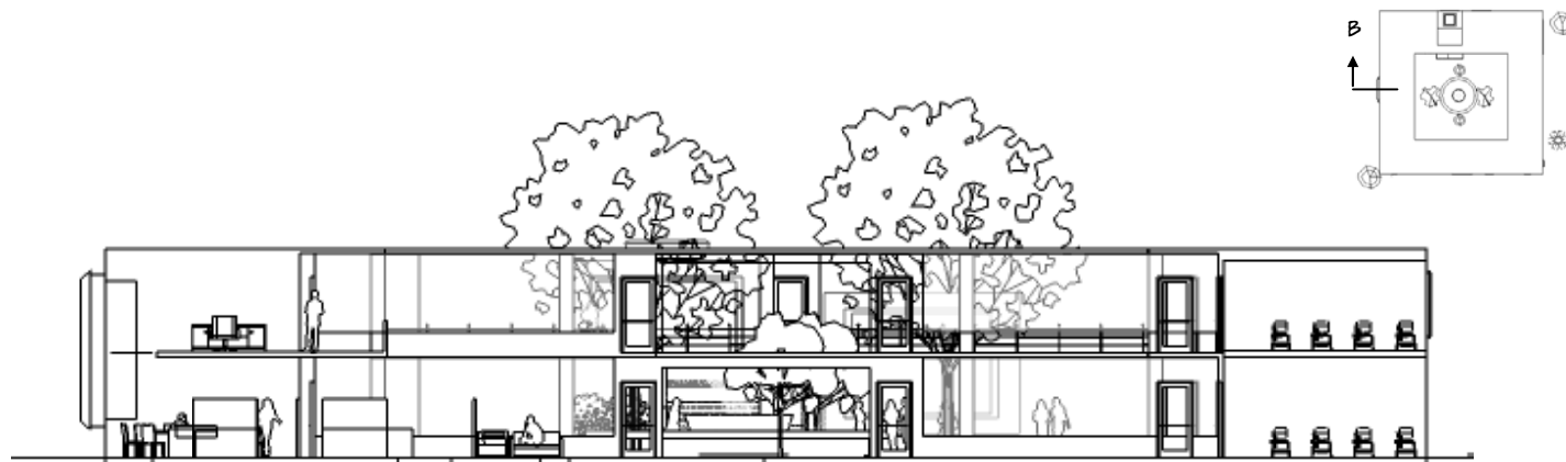
SECCIÓN B NOROESTE SUROESTE
