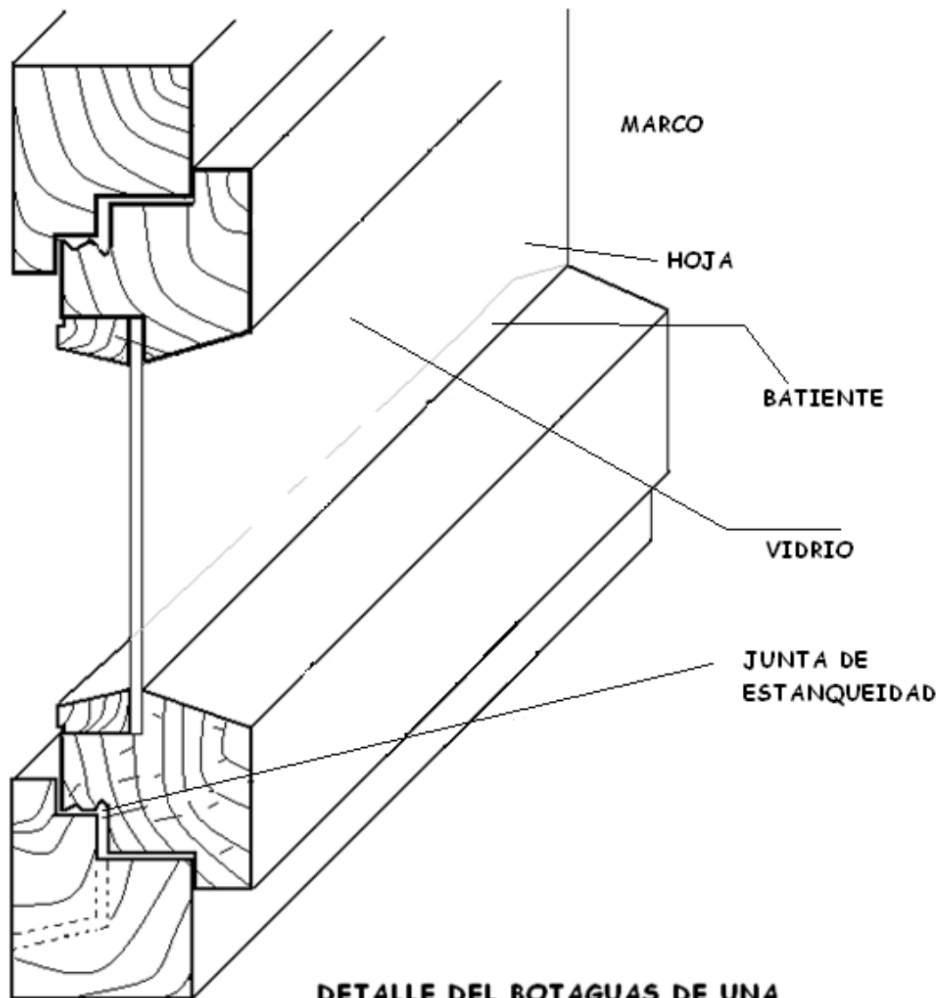
DETALLE DEL BOTAGUAS DE UNA VENTANA DE MADERA
