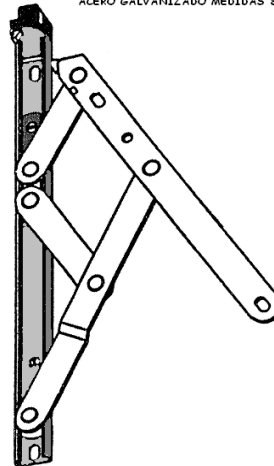
BISAGRA DE FRICCIÓN PARA VENTANA PROYECTABLE DE ACERO GALVANIZADO MEDIDAS 8" 10" 12" 18"
