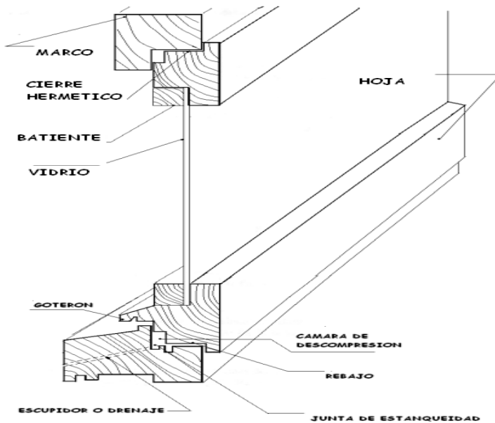
DETALLE DE JUNTA DE ESTANQUEIDAD
