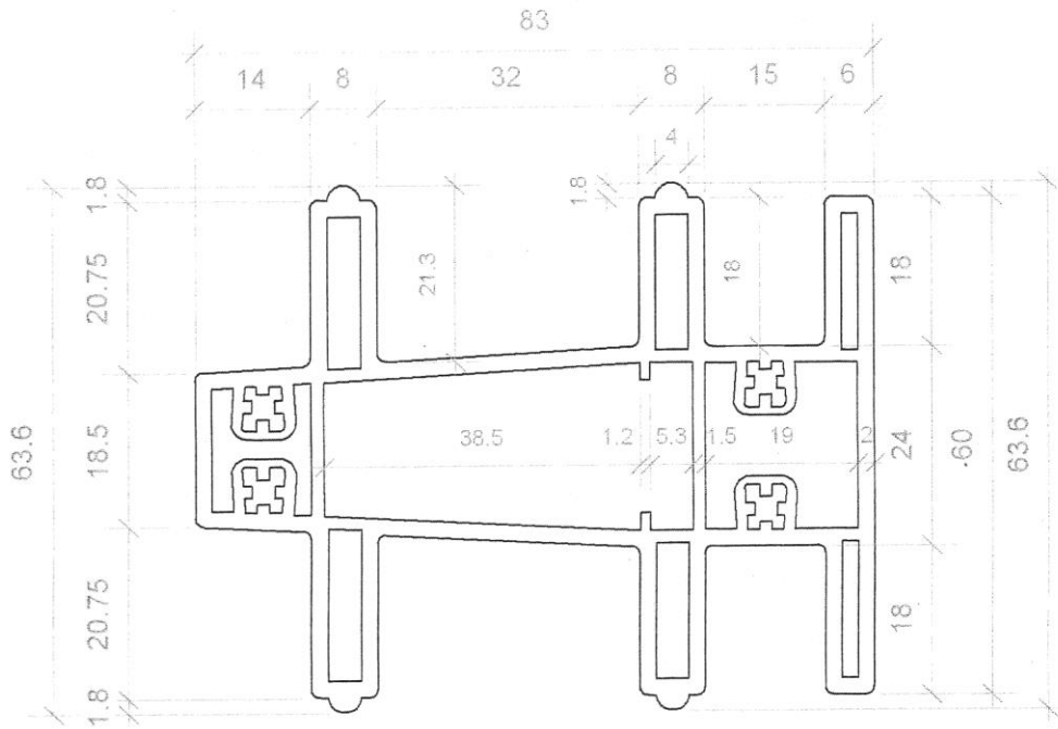
PERFIL A06 INTERMEDIO PARA VENTANAS COMBINADAS
