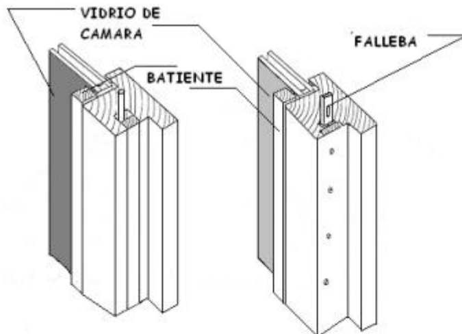
DISTINTAS FORMAS DE COLOCACION DE LA FALLEBA (REFUERZO)
