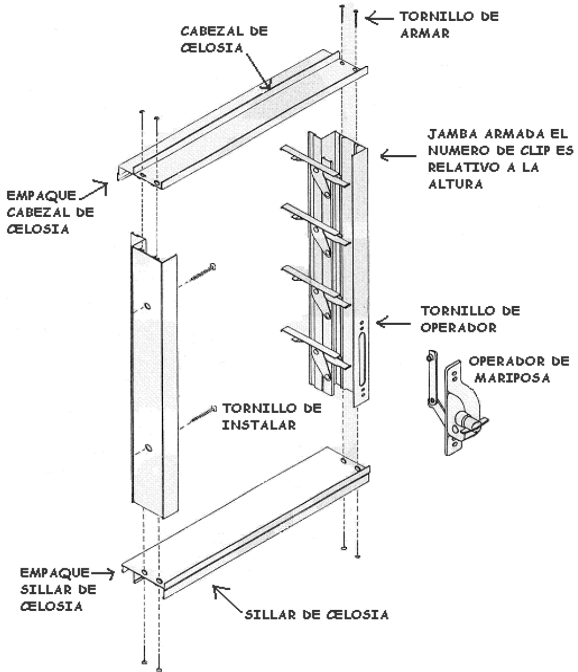
Figura no.25 CELOSÍA ESTANDAR DETALLE DE ARMADO
