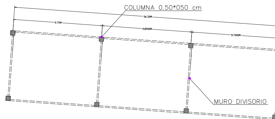
ESTRUCTURA ÁREA DE AULAS Y LABORATORIOS
