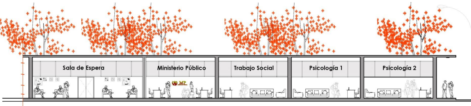
SECCIÓN LONGITUDINAL ÁREA AYUDA INTEGRAL
