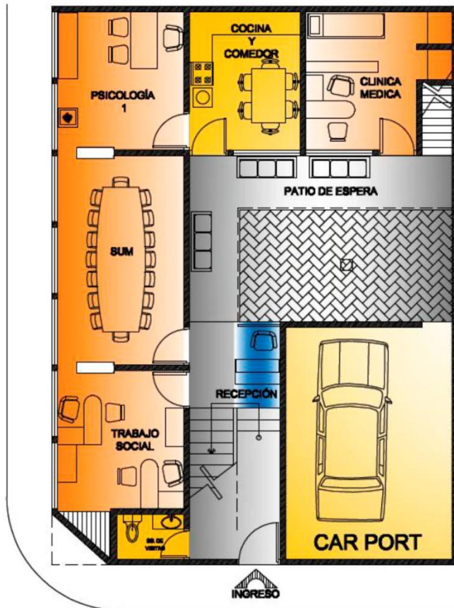
PLANTA CAIMUS 1ER NIVEL
