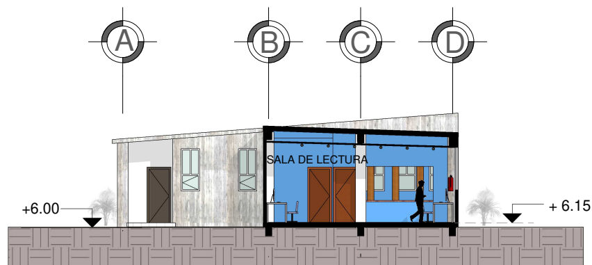
3 Corte Transversal B - B'
