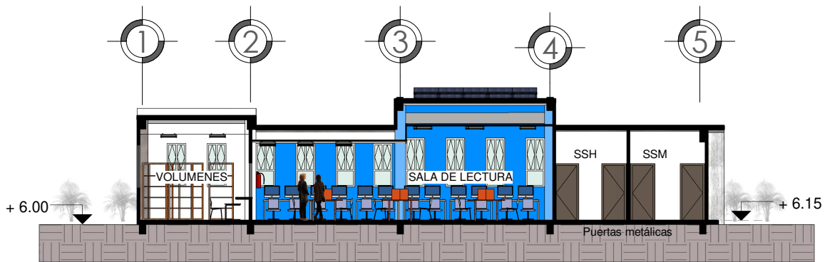
2 Corte Longitudinal A - A'
