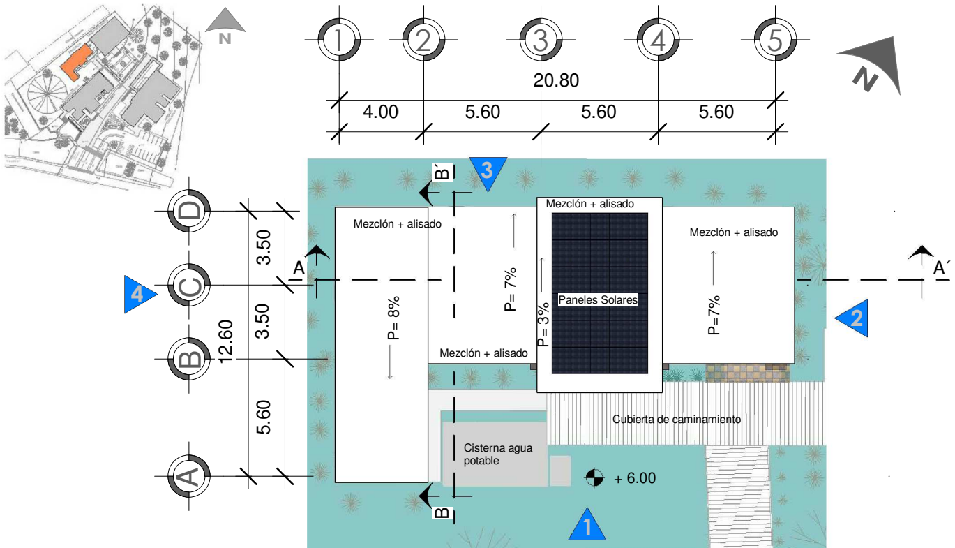
1) Planta de techos - Biblioteca
