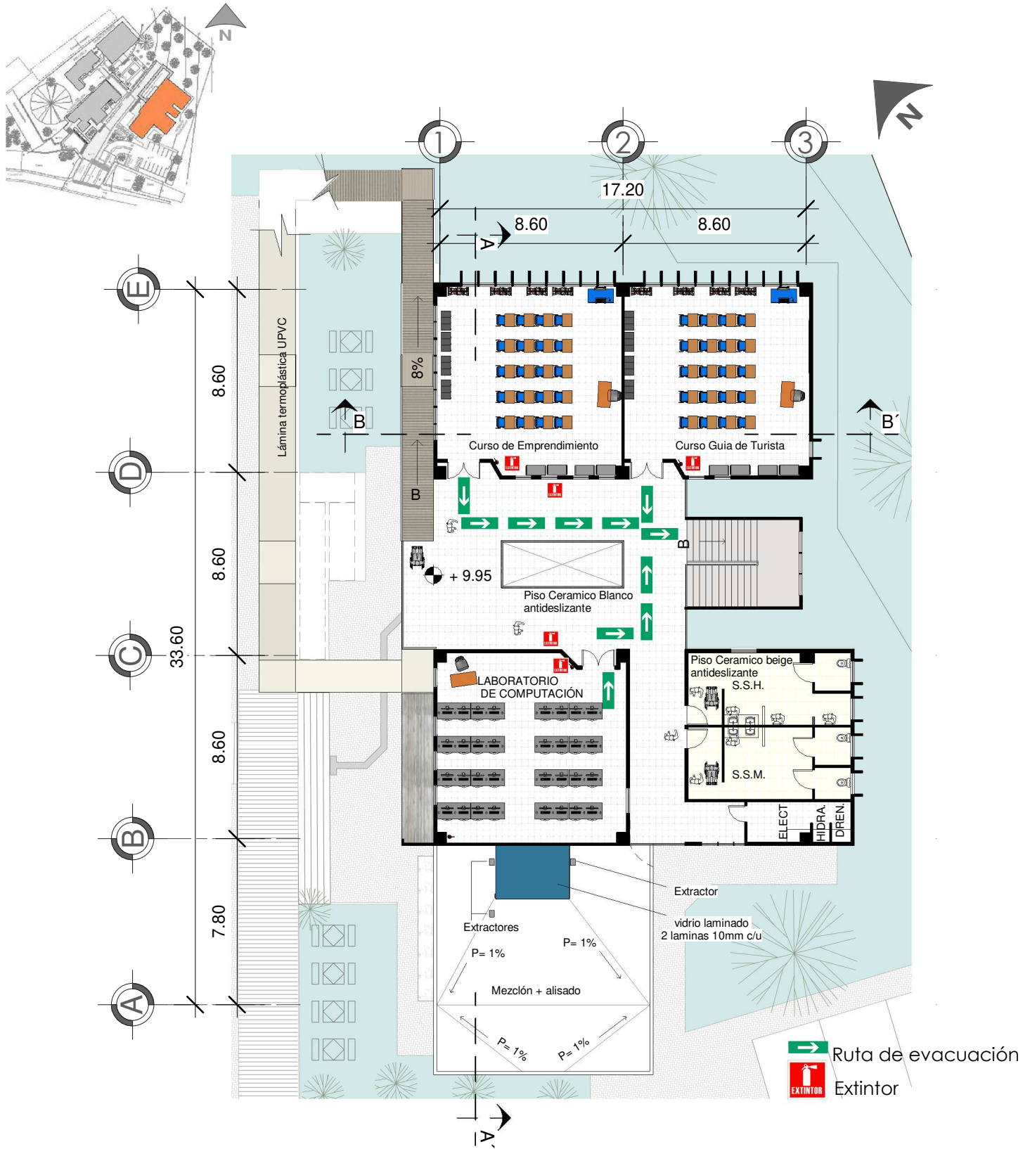
1 Tercer Piso. Módulo educativo
