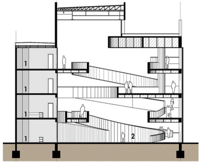
Figura 21. Corte Transversal, Fuente: https://www.plataformaarquitectura.cl/cl/02-342954/instituto-profesional-santo-tomas .
