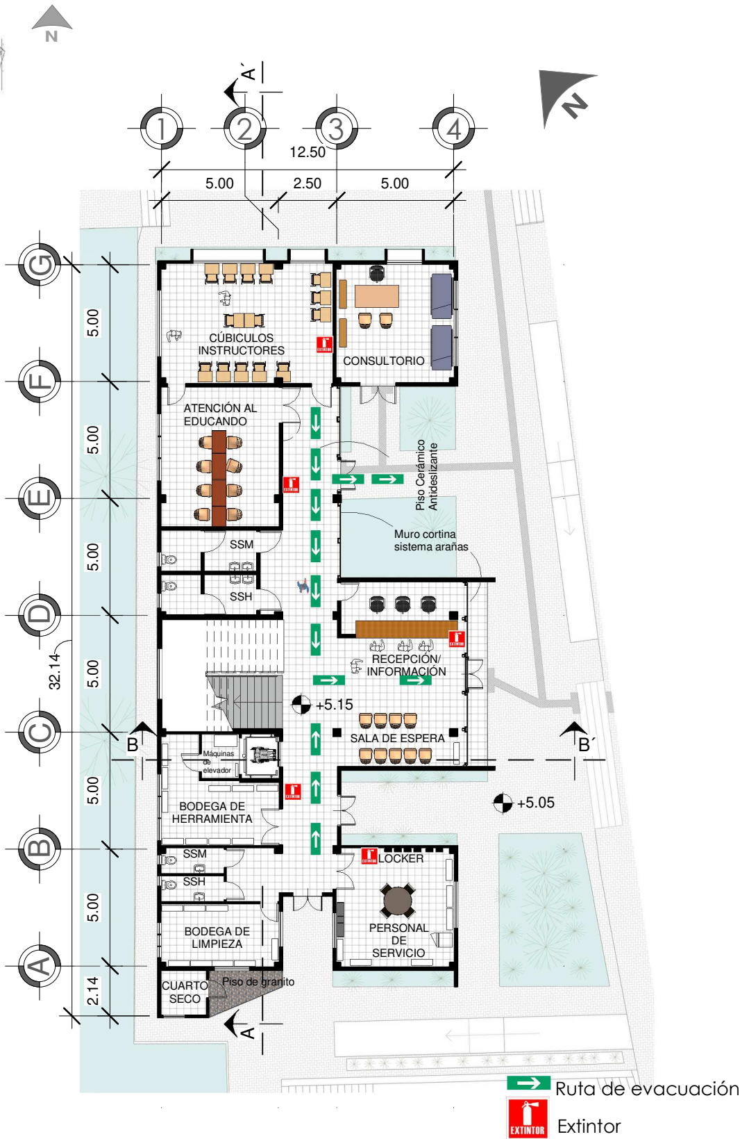
1 Primer Piso. Administración
