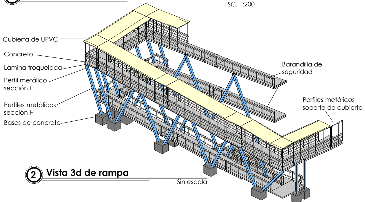
Tramo de rampa del nivel +3.05 al +6.55
