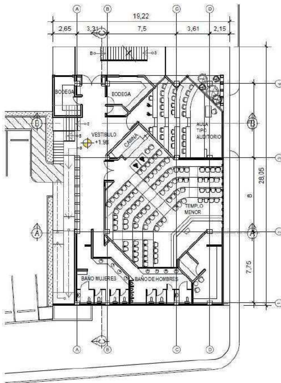
PLANTA ARQUITECTÓNICA Segundo nivel
