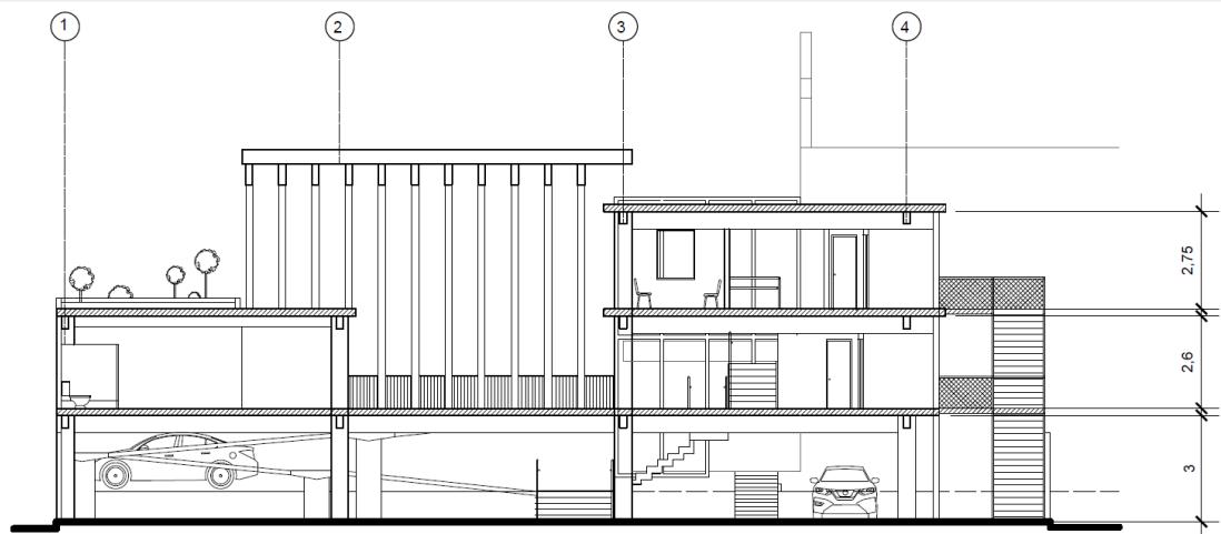
SECCIÓN POR C-C
