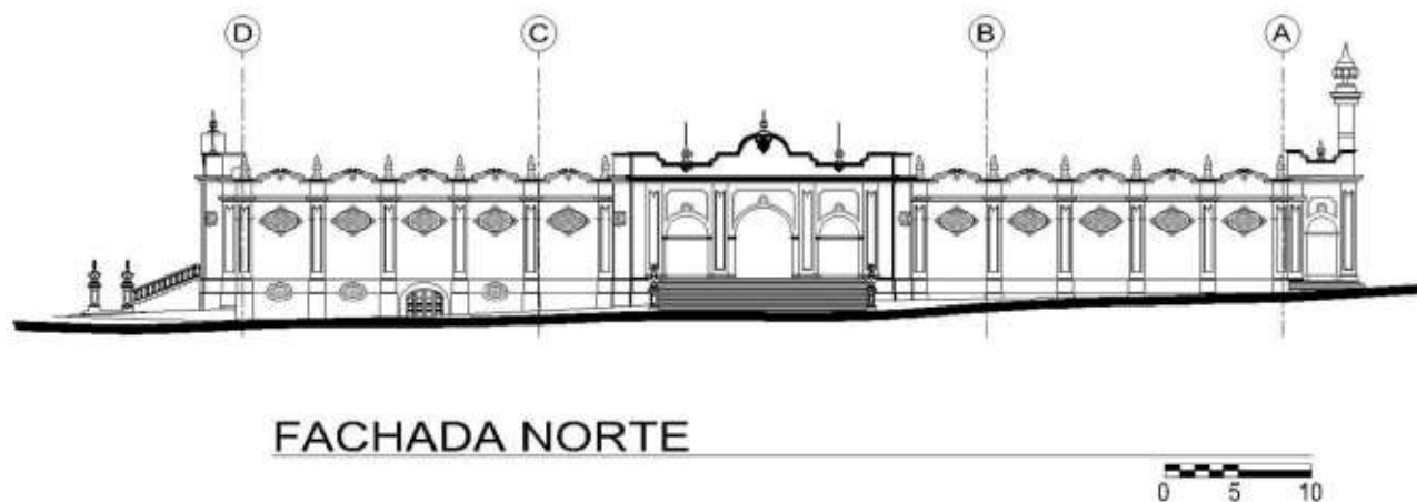
Figura 55 Fachada norte
