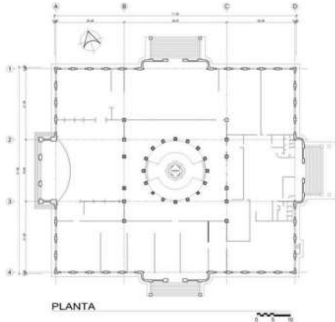
Figura 45 Planta arquitectónica
