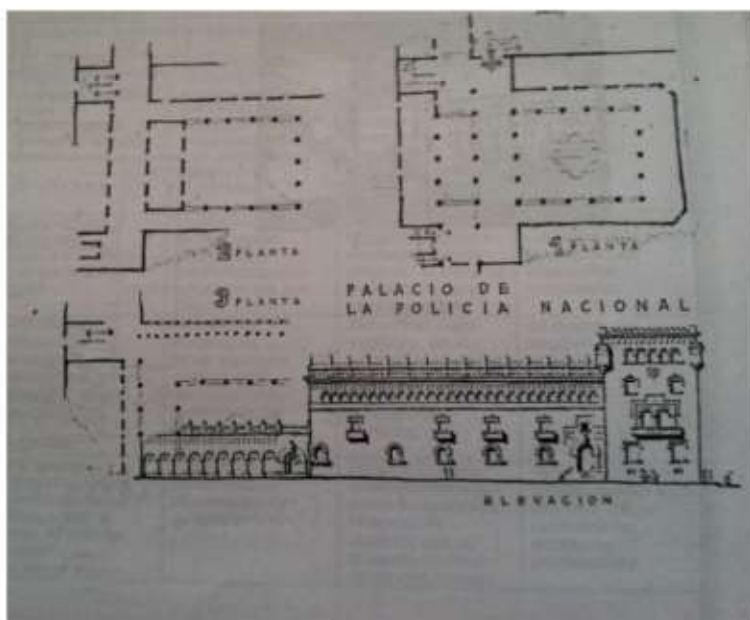
Figura 35 Plano edificio Policía Nacional
